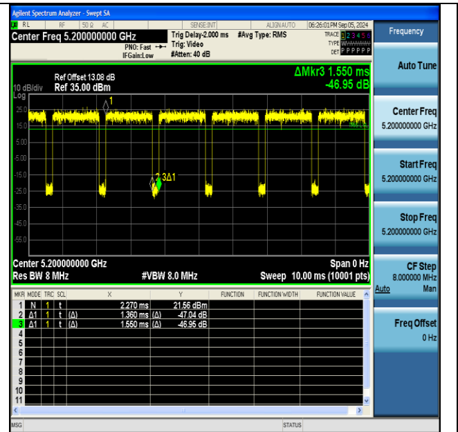
NTVN-11a-Ant1-5200
