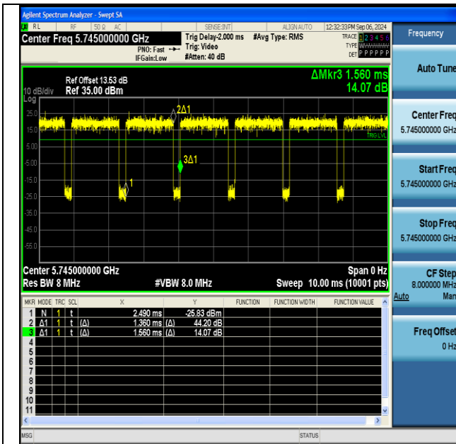
NTNV-11a-Ant1-5745
