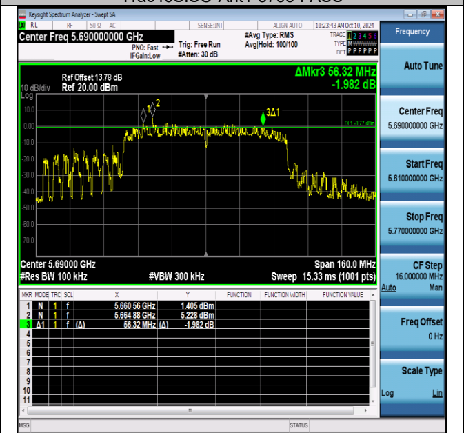
11ac80SISO-Ant1-5690
