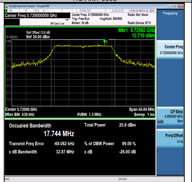
11a-Ant1-5720
