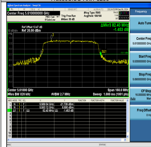
11ac80SISO-Ant1-5610
