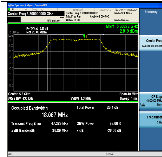
11a-Ant1-5300
