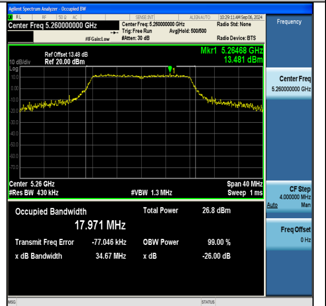
11a-Ant1-5260
