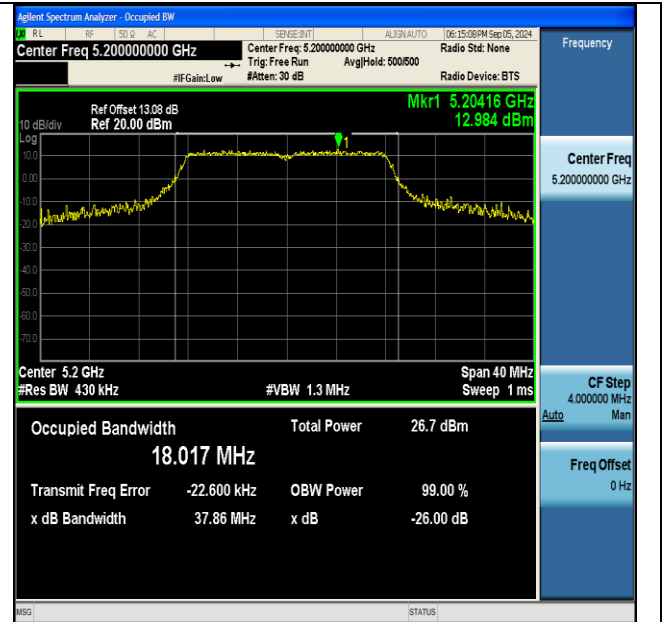
11a-Ant1-5200
