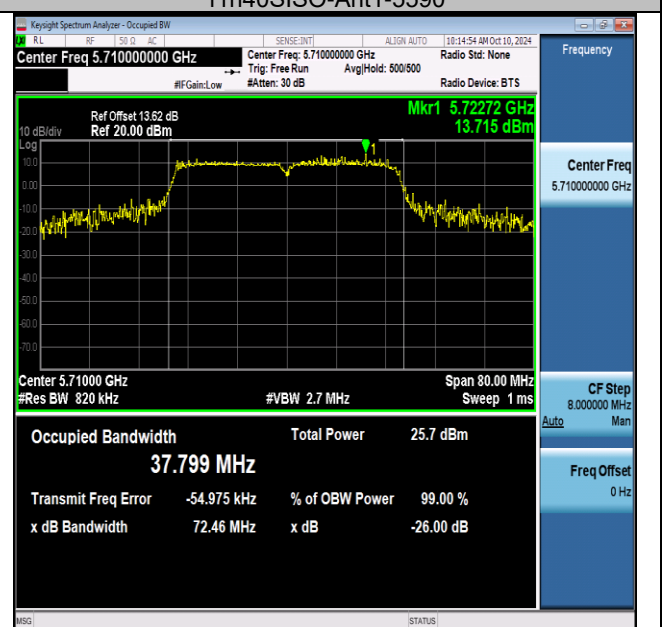
11n40SISO-Ant1-5710
