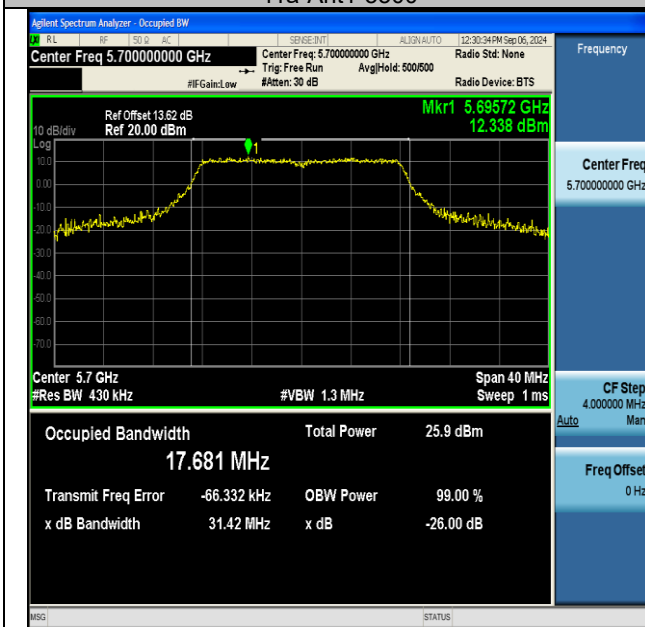
11a-Ant1-5700
