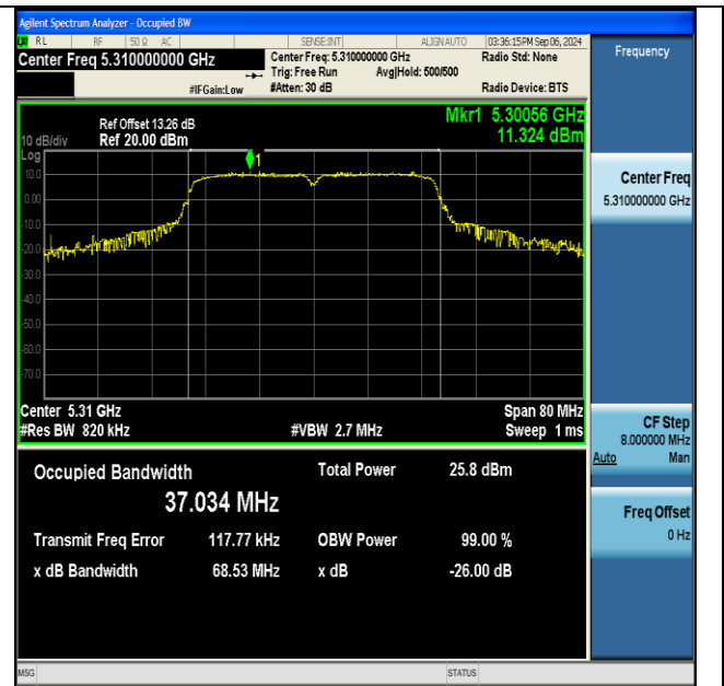
11n40SISO-Ant1-5310
