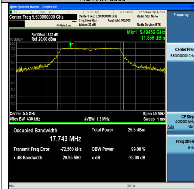
11a-Ant1-5500
