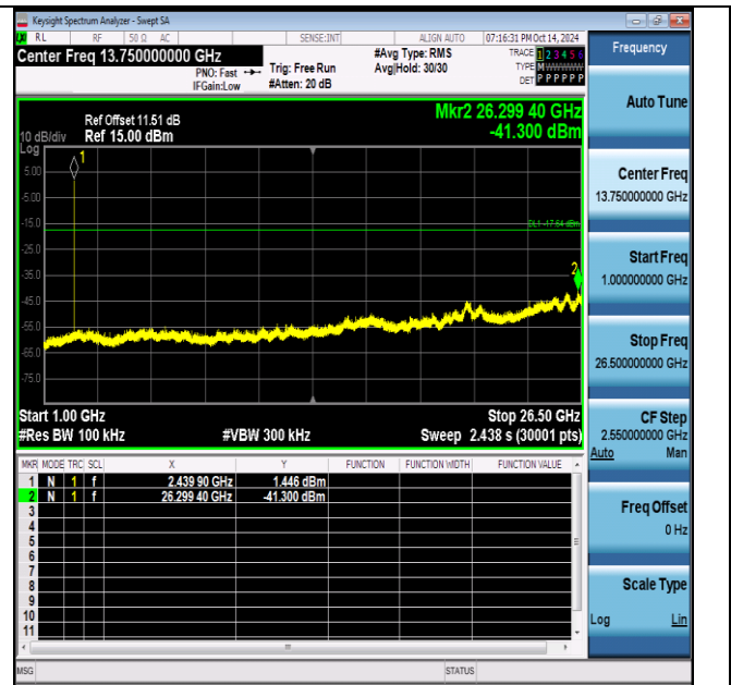
BLE 1M-Ant1-2440-1000~26500-PASS
