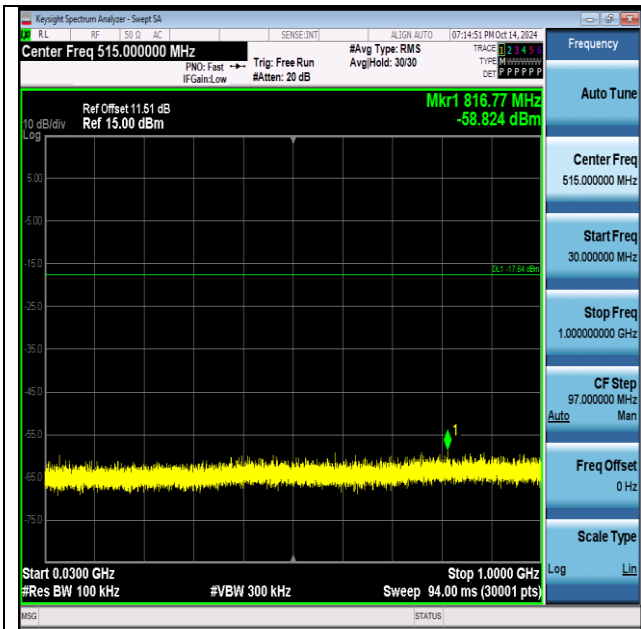
BLE 1M-Ant1-2440-30~1000-PASS
