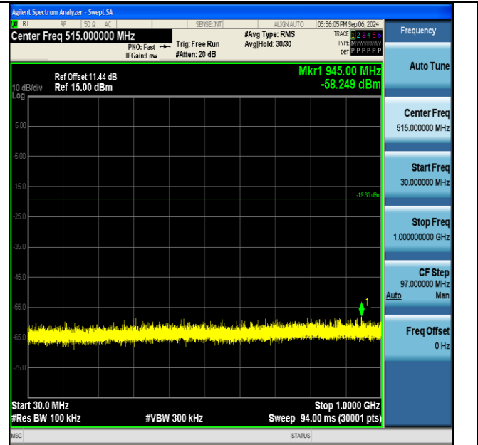
BLE 1M-Ant1-2402-30~1000-PASS
