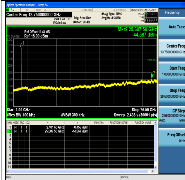
BLE 1M-Ant1-2402-1000~26500-PASS
