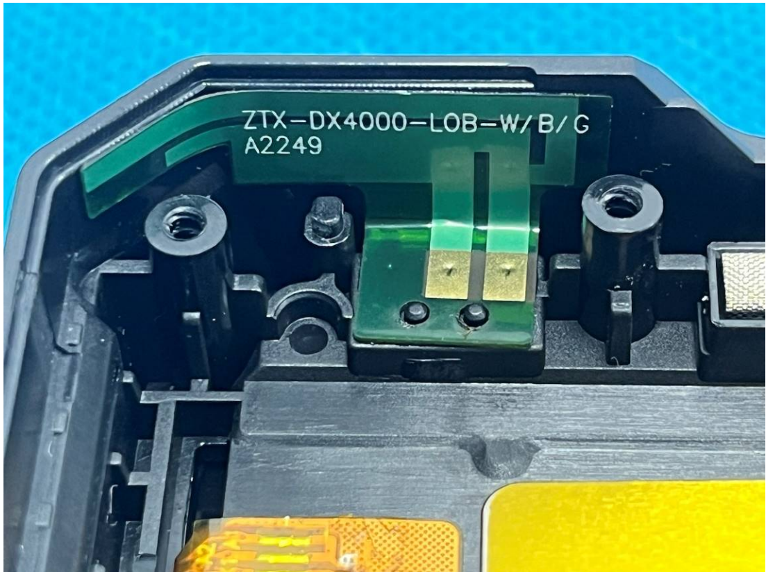
BT/WiFi/GPS Antenna
