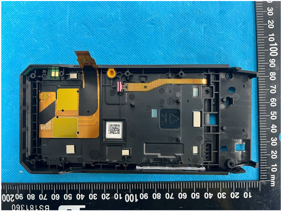
BT/WiFi/GPS Antenna
