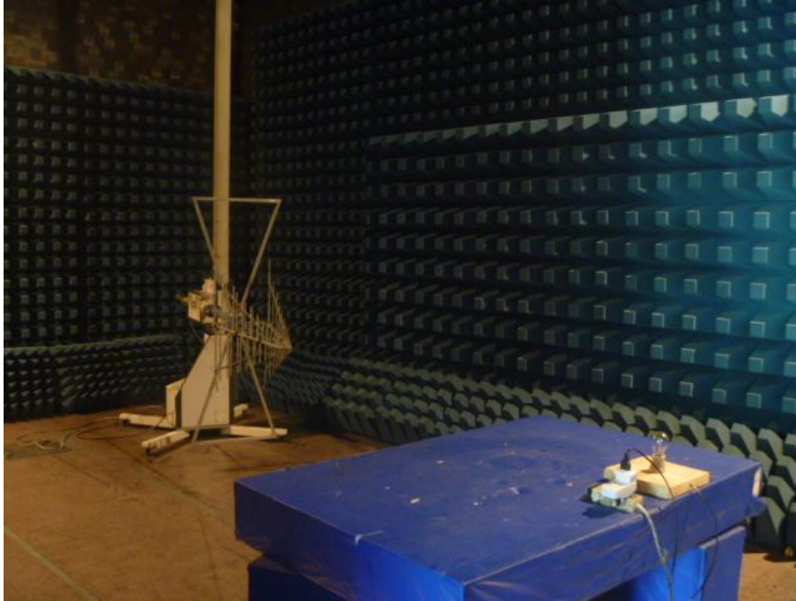
30-1000MHz
