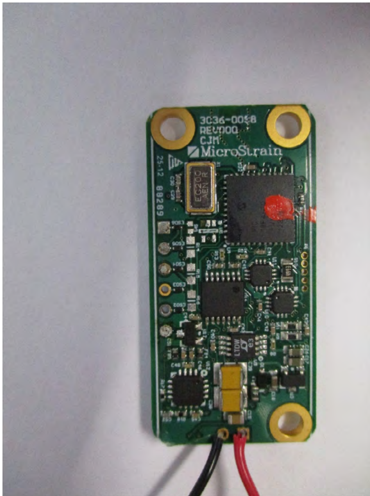
PCB Bottom
