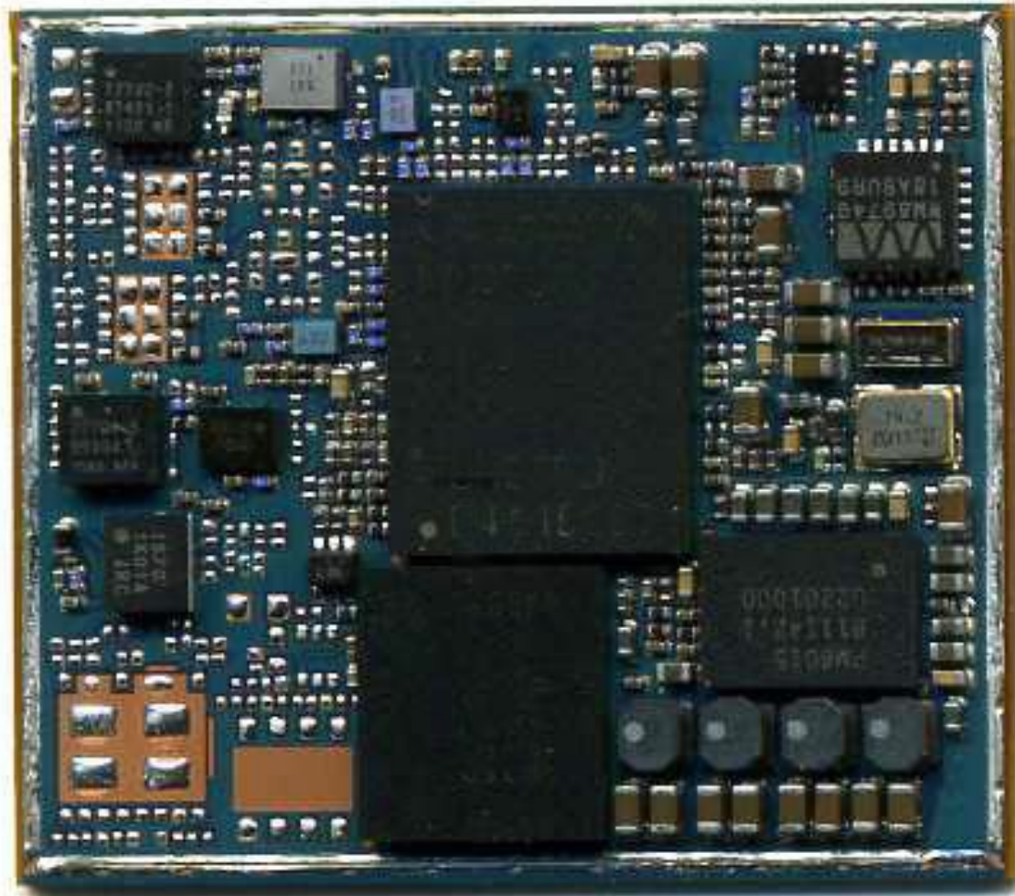
PVS8 Top side
