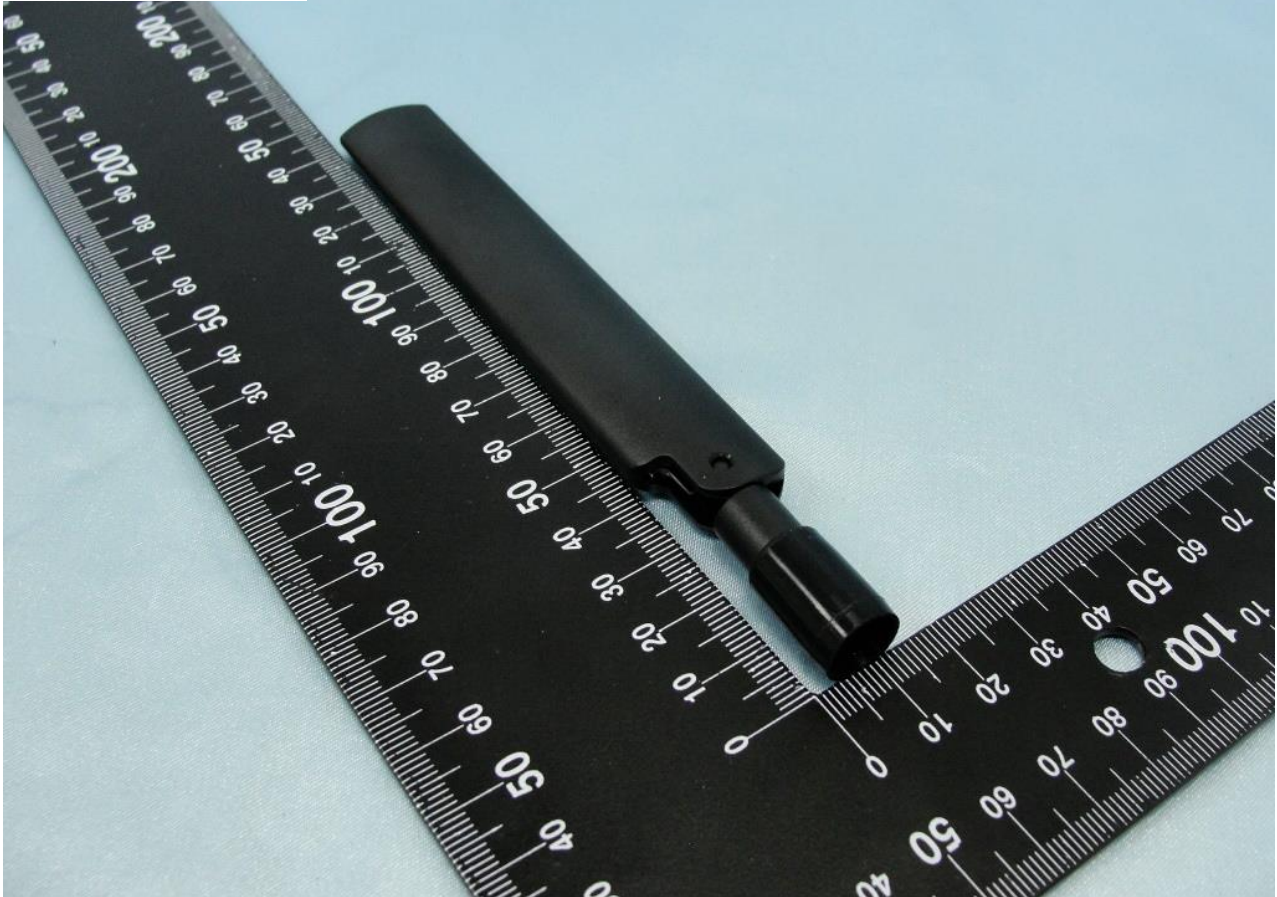
WWAN Antenna 1
