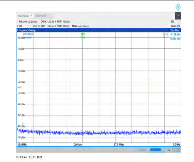
1-N70-PC3-15-15-M-1-DFT-PI2BPSK-Inner_1RB_Le ft-1@1-30-1000-Ant1-66.86--61.19--23-PASS
