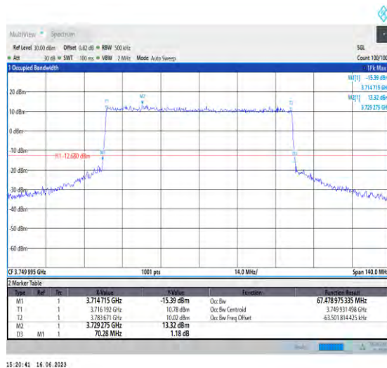
1-N78-3700-3800-PC1-30-70-M-6-CP-QPSK-Outer_Full-189@0-Ant1-67.479-70.280-≤70-PASS
