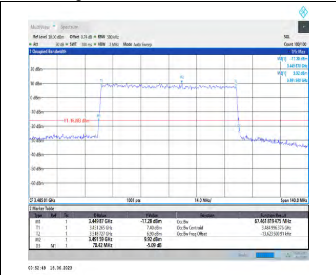
1-N78-3450-3550-PC1.5-30-70-L-9-CP-256QAM-Outer_Full-189@0-Ant1-67.462-70.420-≤70-PASS
