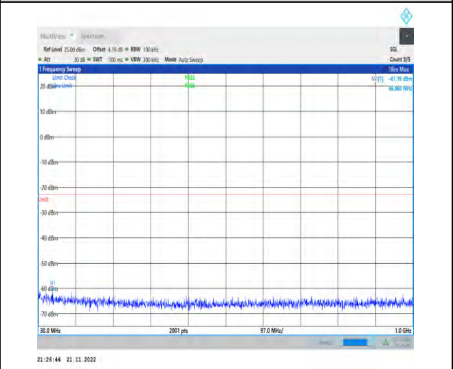
1-N70-PC3-15-15-M-1-DFT-PI2BPSK-Inner_1RB_Le ft-1@1-30-1000-Ant1-66.86--61.19--23-PASS
