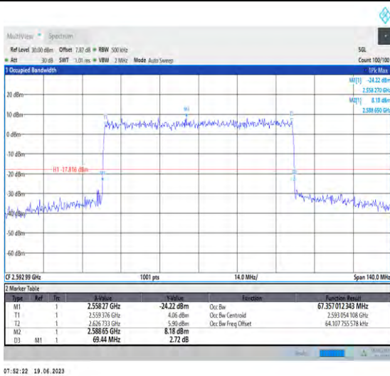
1-N41-PC1.5-30-70-M-9-CP-256QAM-Outer_Full-18 9@0-Ant1-67.357-69.440-≤70-PASS
