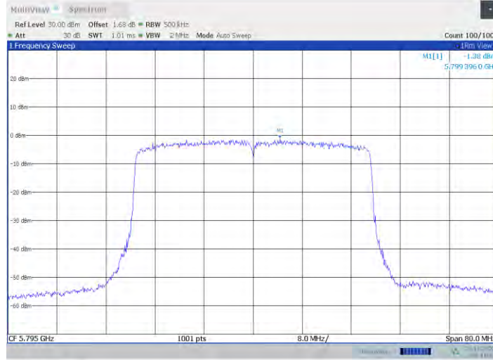
11x40MIMO Ant4 5795
