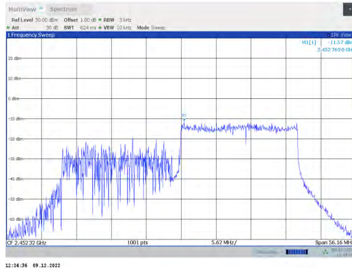
11ax40MIMO_Ant2_2452_106RU+26RU+106R_Right
