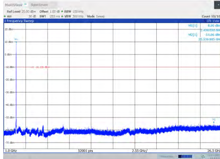
11b-CDD_Ant2_2437_1000~26500
