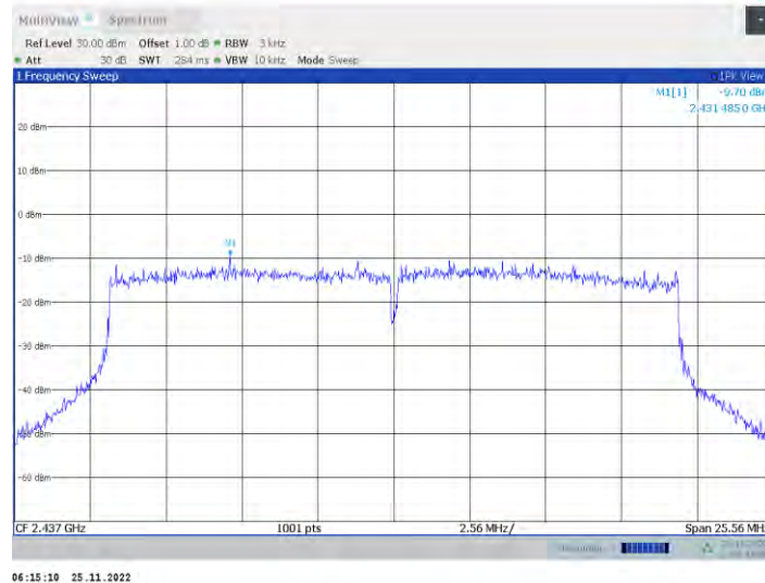
11ax20MIMO_Ant2_2437
