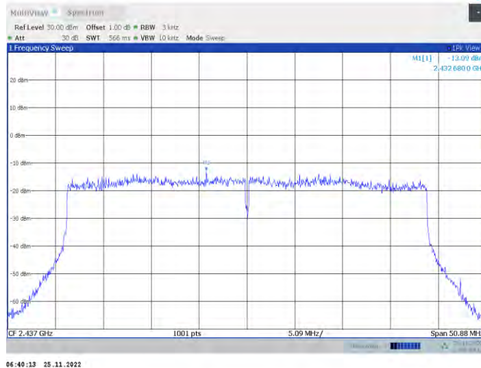
11ax40MIMO_Ant2_2437
