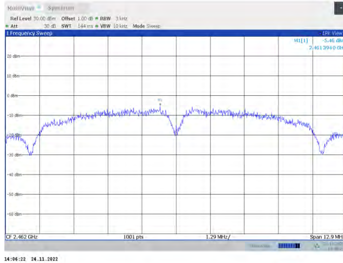
11b-CDD_Ant2_2462
