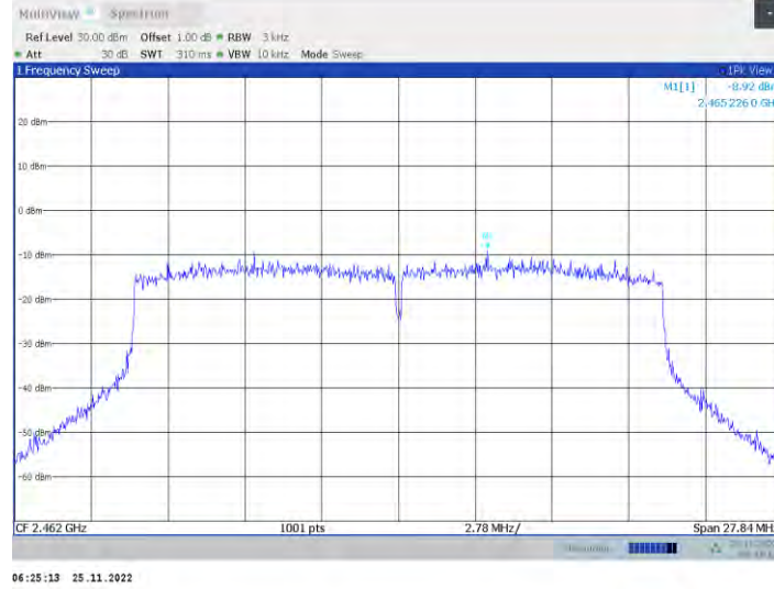
11ax20MIMO_Ant2_2462
