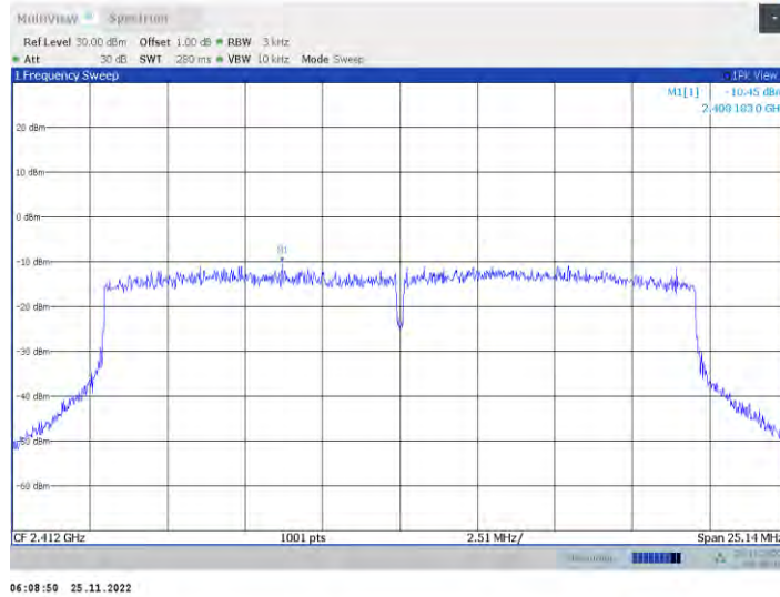
11ax20MIMO_Ant2_2412
