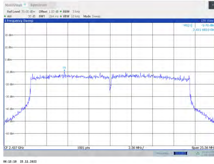
11ax20MIMO_Ant2_2437
