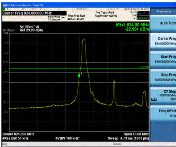
LTE Band 5 QPSK 5MHz CH-Low 1RB
