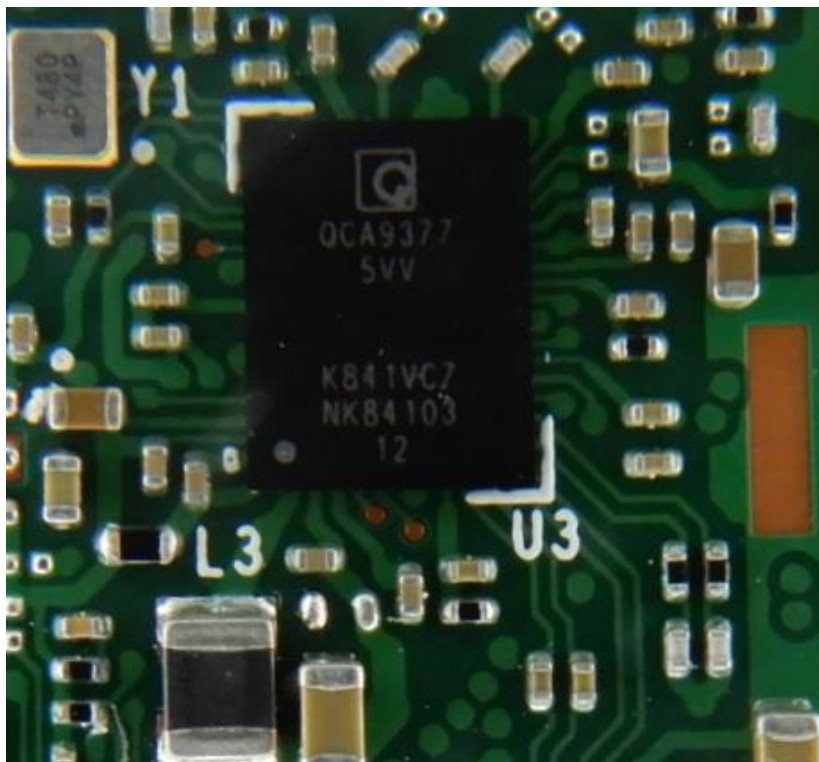
RF IC
