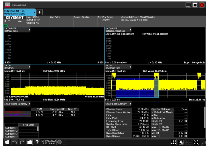
n2_20MHz_15kHz_1880MHz_DFT-s-OFDM QPSK_RB100@0
