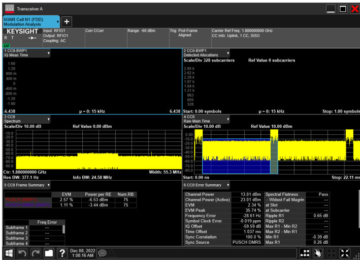
n2_15MHz_15kHz_1880MHz_DFT-s-OFDM QPSK_RB75@0
