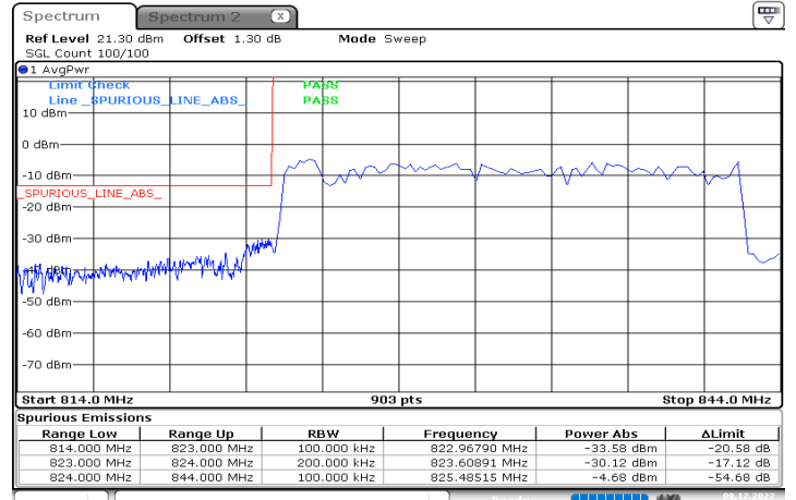
n5_20MHz_15kHz_834MHz_DFT-s-OFDM QPSK_RB100@0
