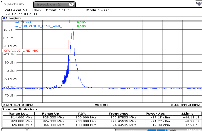
n5_20MHz_15kHz_834MHz_DFT-s-OFDM QPSK_RB1@0
