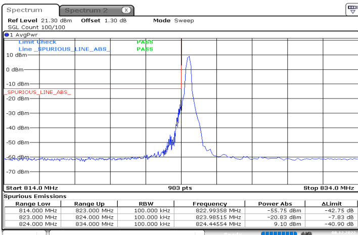
n5_10MHz_15kHz_829MHz_DFT-s-OFDM QPSK_RB1@0
