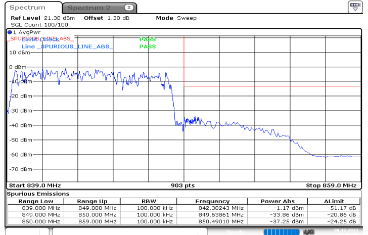
n5_10MHz_15kHz_844MHz_DFT-s-OFDM QPSK_RB50@0
