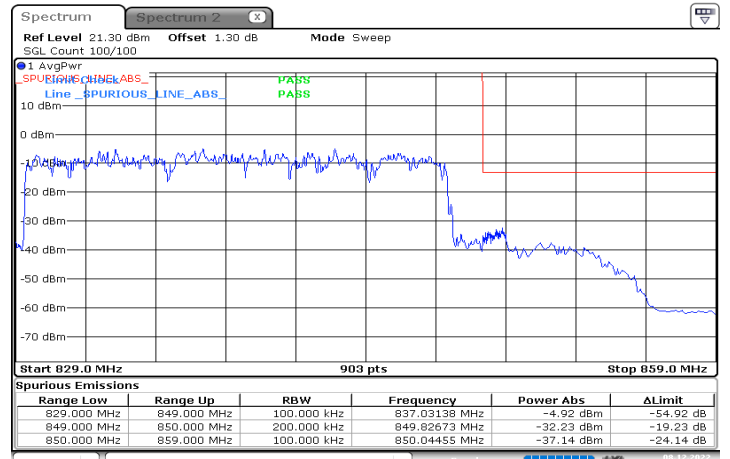
n5_20MHz_15kHz_839MHz_DFT-s-OFDM QPSK_RB100@105
