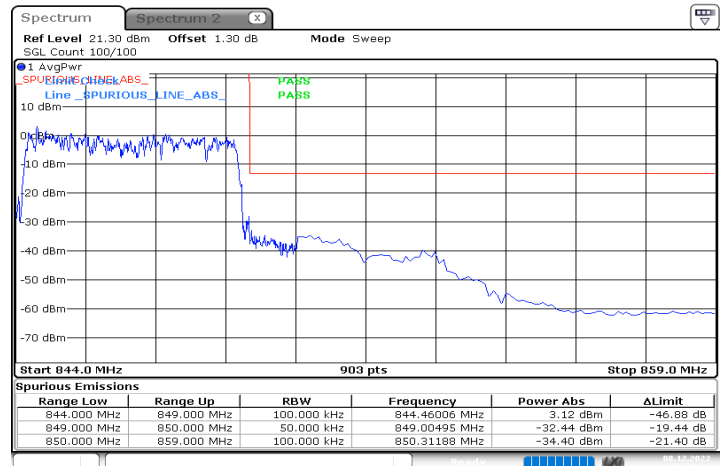
n5_5MHz_15kHz_846.5MHz_DFT-s-OFDM QPSK_RB25@0
