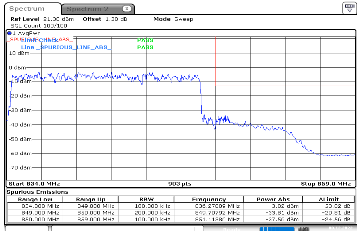
n5_15MHz_15kHz_841.5MHz_DFT-s-OFDM QPSK_RB75@0
