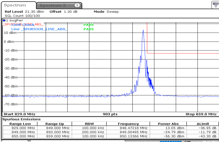
n5_20MHz_15kHz_839MHz_DFT-s-OFDM QPSK_RB1@105
