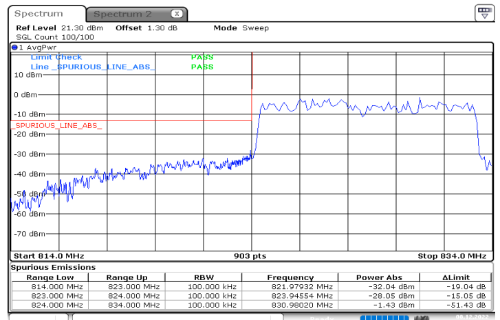
n5_10MHz_15kHz_829MHz_DFT-s-OFDM QPSK_RB50@0
