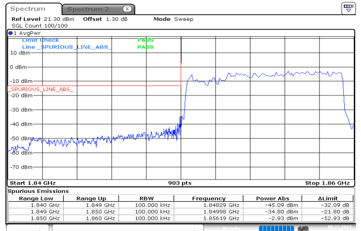
n2_10MHz_15kHz_1855MHz_DFT-s-OFDM QPSK_RB50@0
