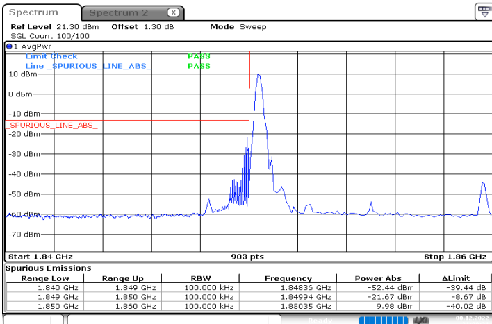
n2_10MHz_15kHz_1855MHz_DFT-s-OFDM QPSK_RB1@0
