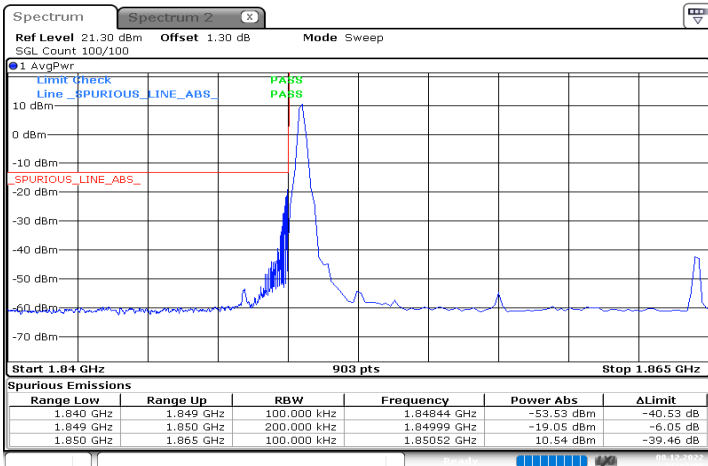
n2_15MHz_15kHz_1857.5MHz_DFT-s-OFDM QPSK_RB1@0
