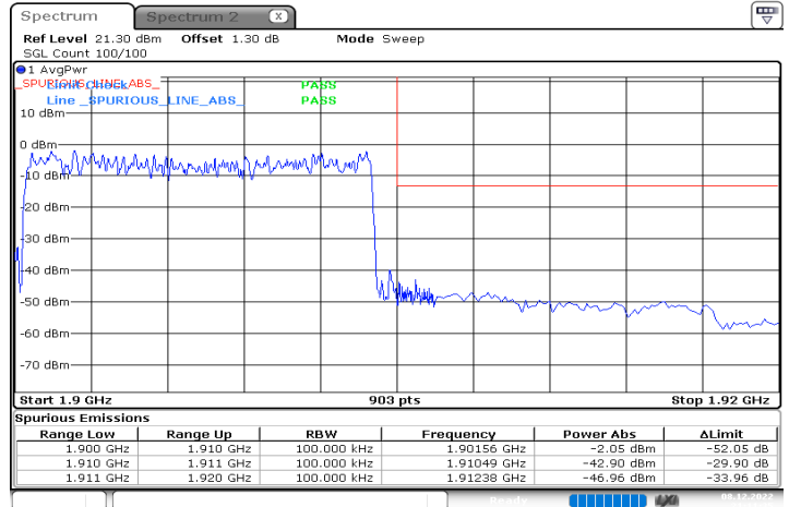
n2_10MHz_15kHz_1905MHz_DFT-s-OFDM QPSK_RB50@0
