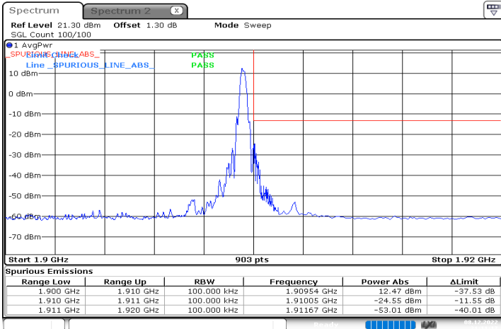
n2_10MHz_15kHz_1905MHz_DFT-s-OFDM QPSK_RB1@51
