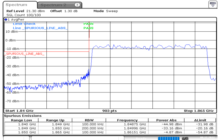
n2_15MHz_15kHz_1857.5MHz_DFT-s-OFDM QPSK_RB75@0
