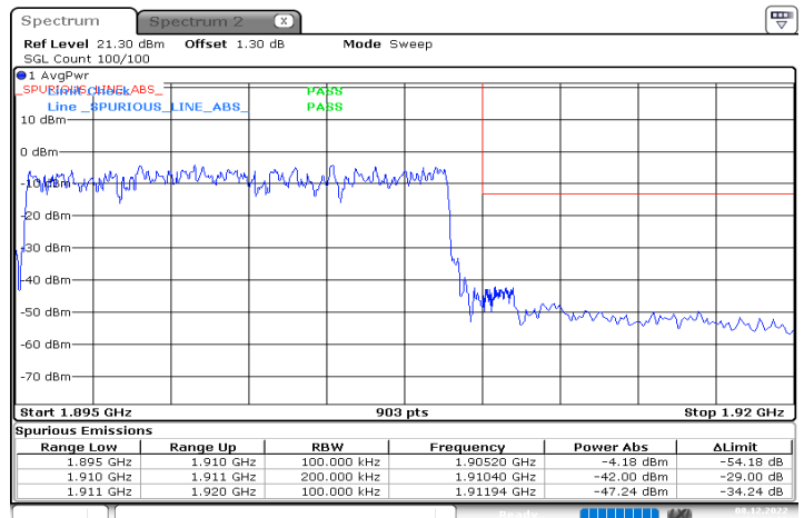
n2_15MHz_15kHz_1902.5MHz_DFT-s-OFDM QPSK_RB75@0
