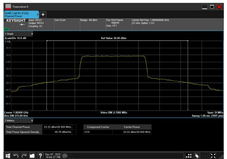
n2_20MHz_15kHz_1860MHz_DFT-s-OFDM QPSK_RB50@25
