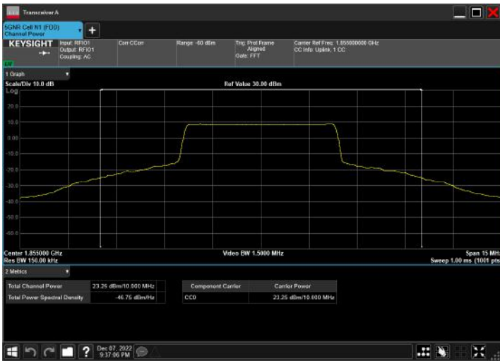
n2_10MHz_15kHz_1855MHz_CP-OFDM QPSK_RB52@0
