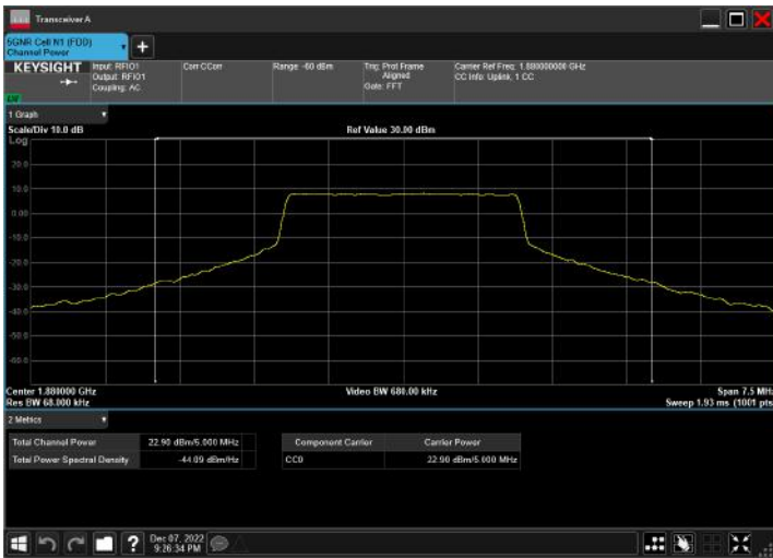
n2_5MHz_15kHz_1880MHz_CP-OFDM QPSK_RB25@0
