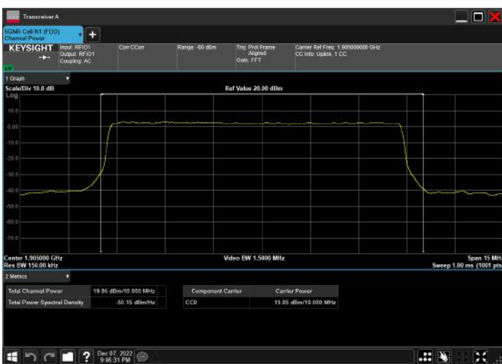
n2_10MHz_15kHz_1905MHz_DFT-s-OFDM 256 QAM_RB50@0
