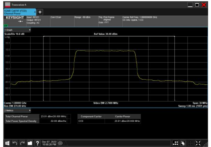
n2_20MHz_15kHz_1880MHz_DFT-s-OFDM PI/2 BPSK_RB50@25
