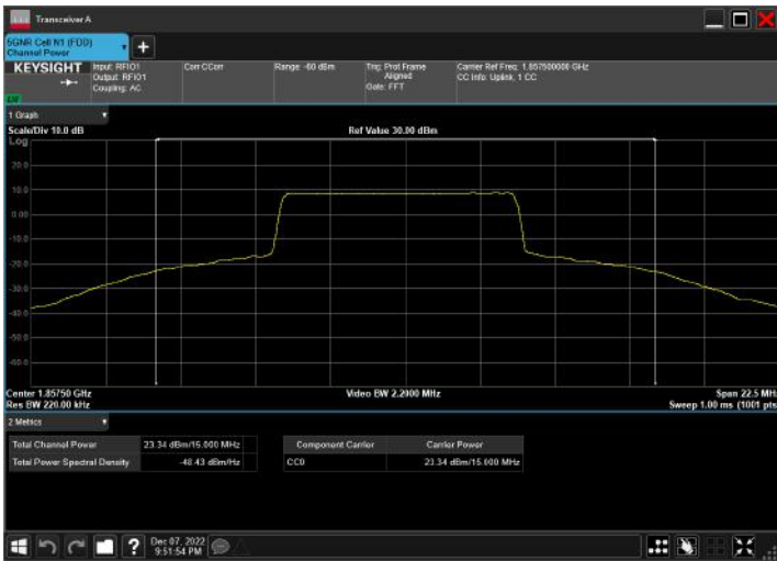
n2_15MHz_15kHz_1857.5MHz_CP-OFDM QPSK_RB79@0
