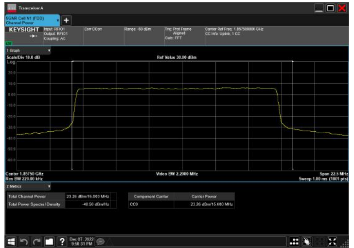
n2_15MHz_15kHz_1857.5MHz_DFT-s-OFDM QPSK_RB75@0
