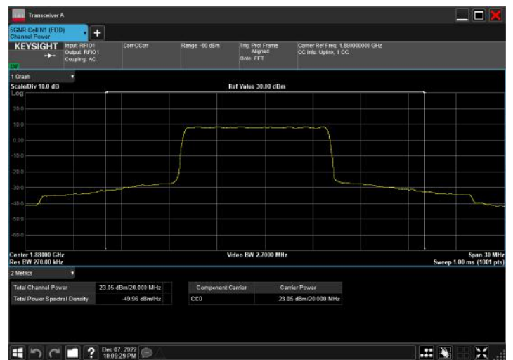
n2_20MHz_15kHz_1880MHz_DFT-s-OFDM QPSK_RB50@25
