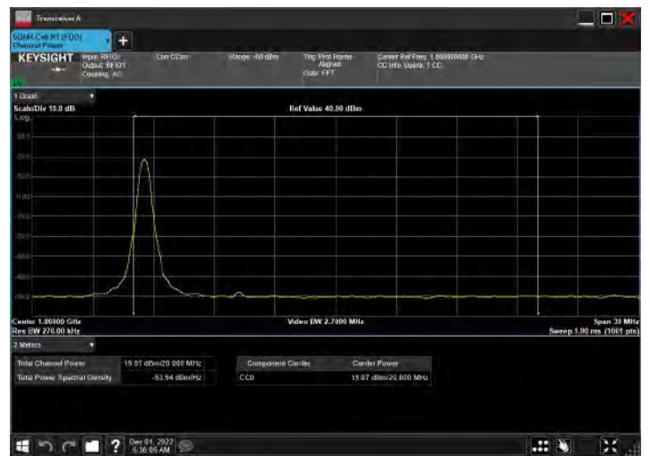
DC_66A_n2A_10MHz|20MHz_15kHz_1715MHz|1860MHz_QPSK|DFT-s-OFDM QPSK_RB1@0|RB1@0
