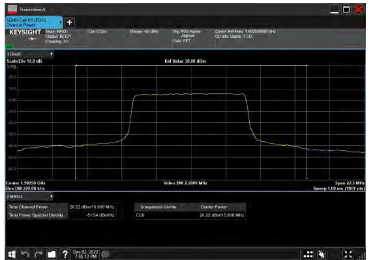
DC_66A_n2A_10MHz|15MHz_15kHz_1775MHz|1902.5MHz_QPSK|CP-OFDM QPSK_RB12@38|RB39@19
