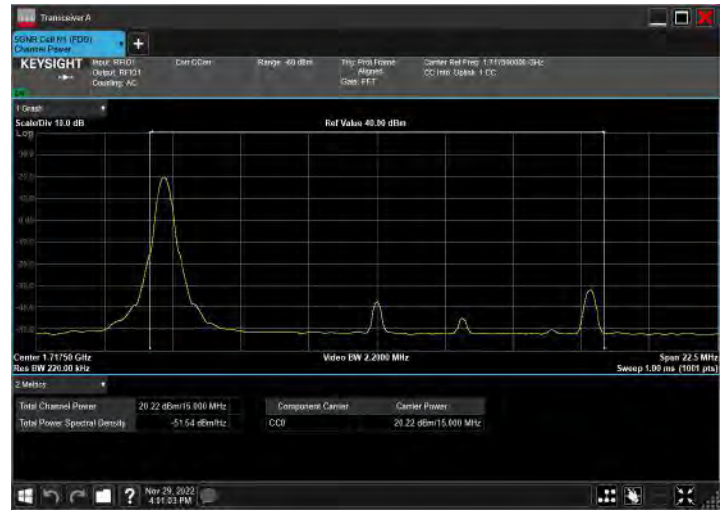
DC_2A_n66A_10MHz|15MHz_15kHz_1855MHz|1717.5MHz_QPSK|CP-OFDM QPSK_RB1@0|RB1@0
