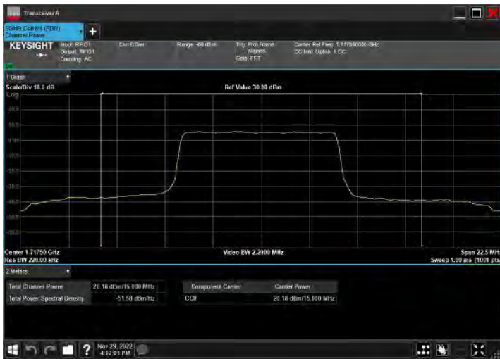
DC_2A_n66A_10MHz|15MHz_15kHz_1855MHz|1717.5MHz_QPSK|CP-OFDM QPSK_RB12@0|RB39@19
