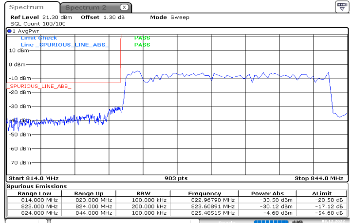
n5_20MHz_15kHz_834MHz_DFT-s-OFDM QPSK_RB100@0
