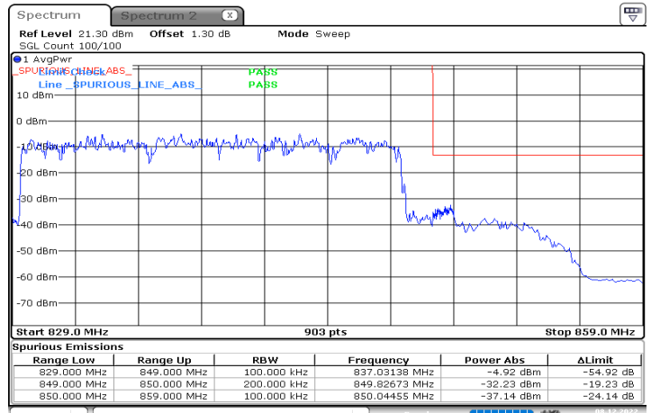
n5_20MHz_15kHz_839MHz_DFT-s-OFDM QPSK_RB100@105
