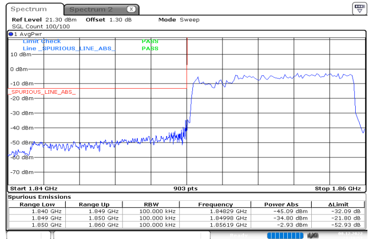
n2_10MHz_15kHz_1855MHz_DFT-s-OFDM QPSK_RB50@0
