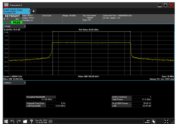
n2_15MHz_15kHz_1880MHz_CP-OFDM QPSK_RB79@0
