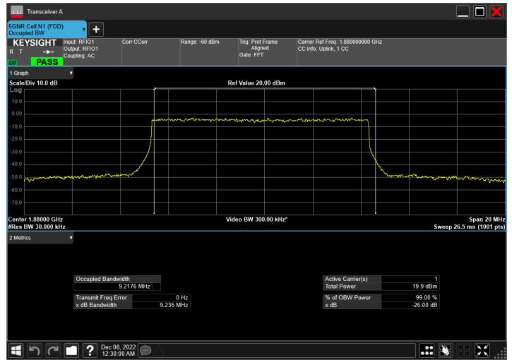
n2_10MHz_15kHz_1880MHz_DFT-s-OFDM 256 QAM_RB50@0
