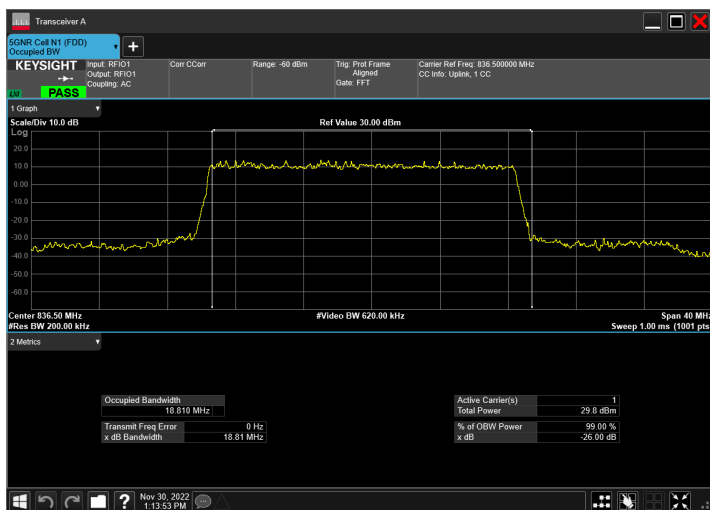
DC_2A_n5A_10MHz|20MHz_15kHz_1880MHz|836.5MHz_QP SK|DFT-s-OFDM PI/2 BPSK_RB1@50|RB100@0
