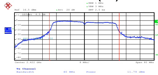
802.11n(H40)
