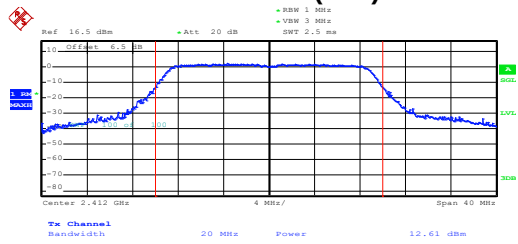
802.11n(H20)
