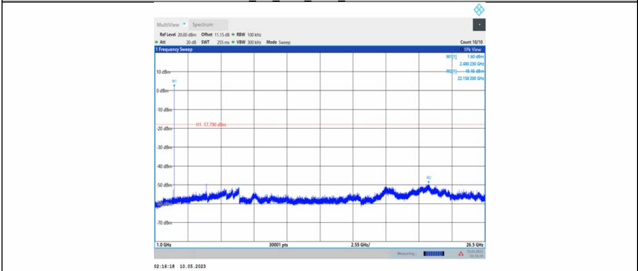
BLE_1M_Ant1_2480_1000~26500
