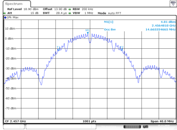
IEEE 802.11b CH10
