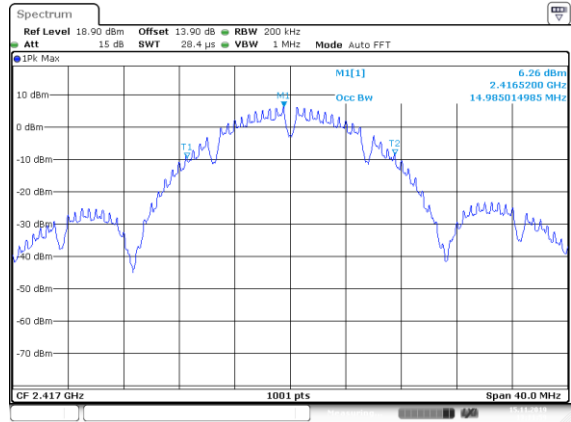
IEEE 802.11b CH2
