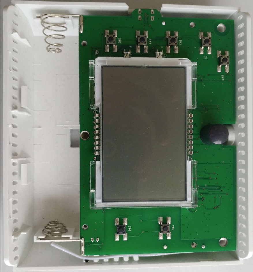
Antenna
