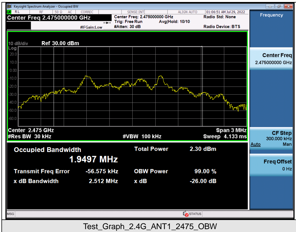
Test_Graph_2.4G_ANT1_2475_OBW
