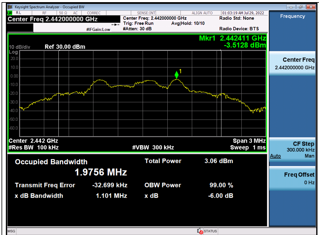
Test_Graph_2.4G_ANT1_2442_DTSBW
