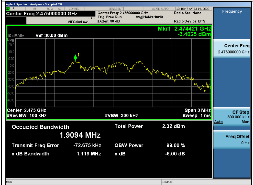
Test_Graph_2.4G_ANT1_2475_DTSBW
