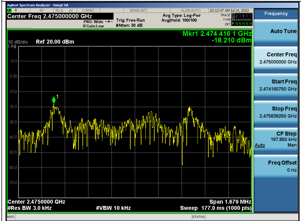
Test_Graph_2.4G_ANT1_2475_PSD
