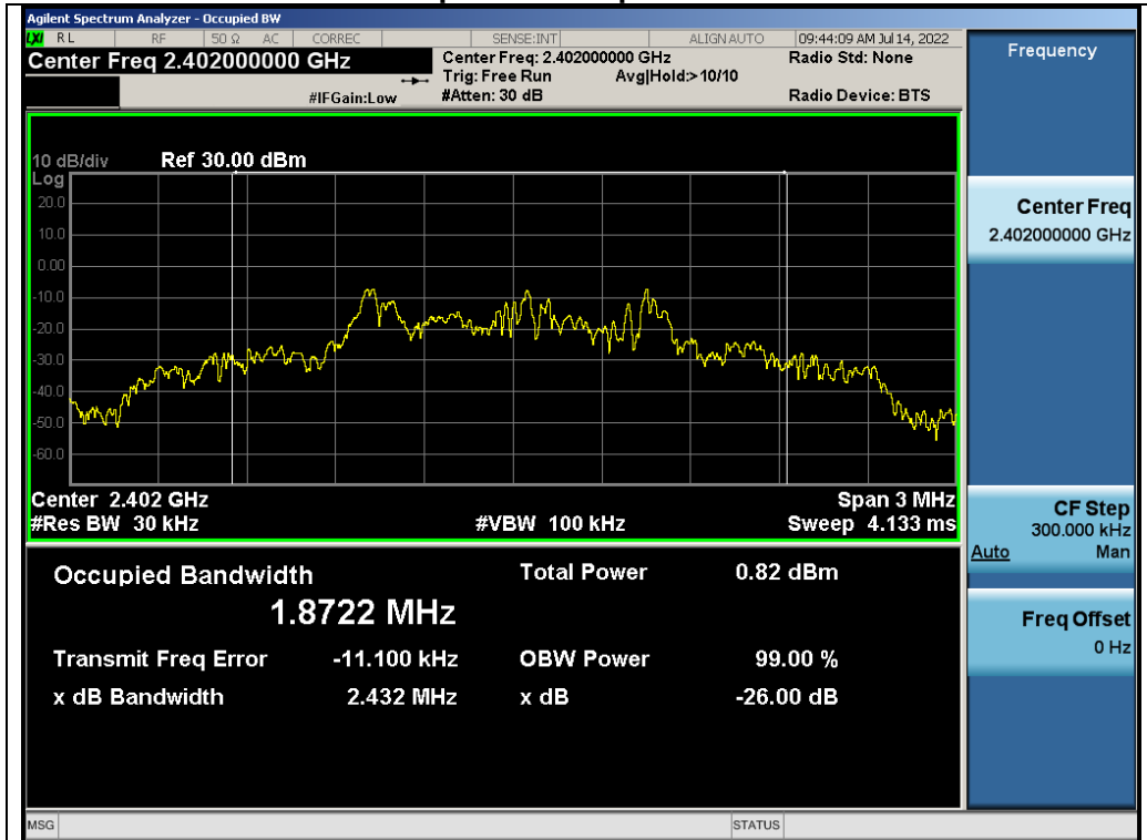
Test_Graph_2.4G_ANT1_2402_OBW
