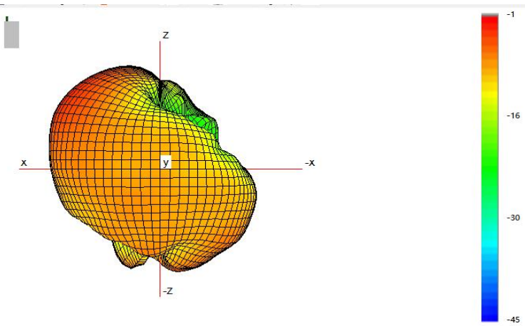
FREQUENCY=2500MHZ
