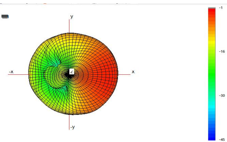
FREQUENCY=2500MHZ
