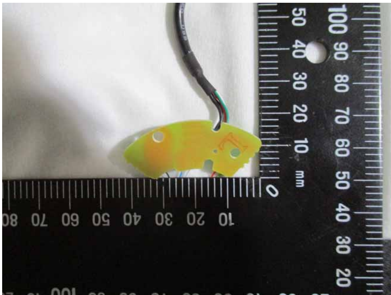
Antenna
