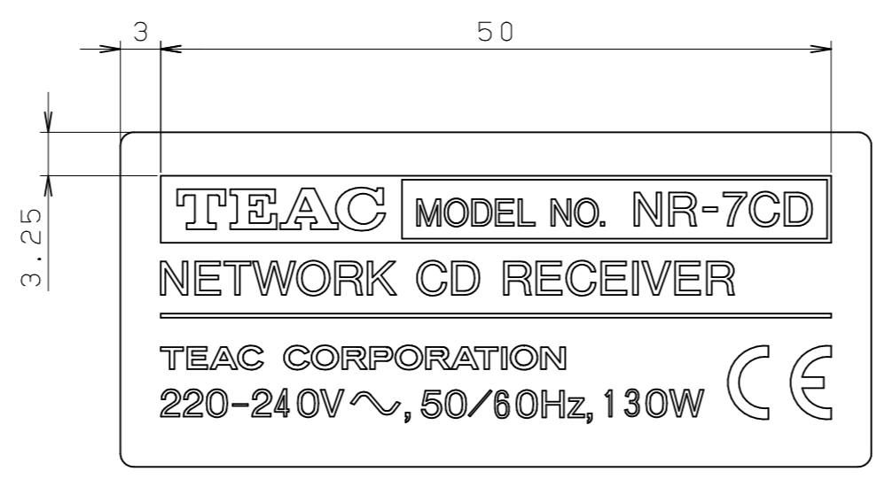
印字位置
