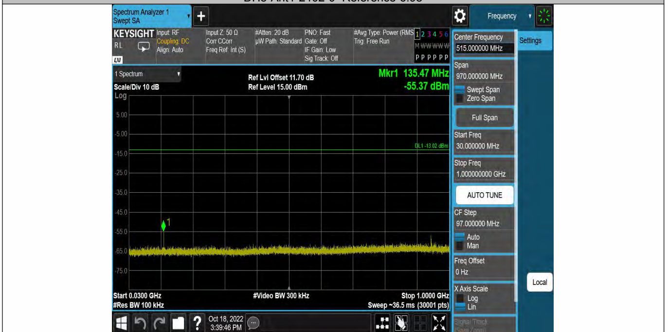
DH5-Ant1-2402-30~1000-6.98
