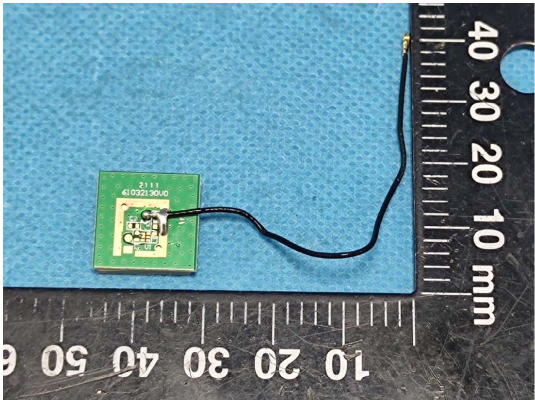
GPS Antenna
