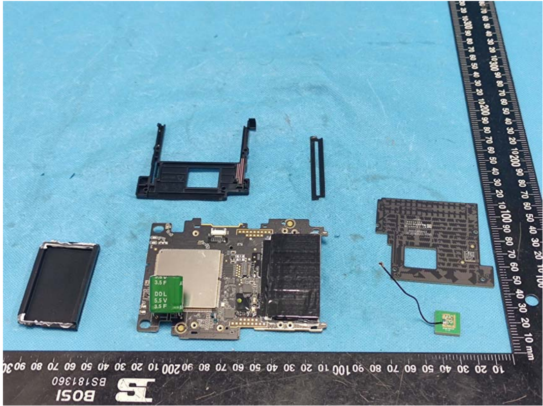
GPS Antenna
