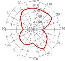
1700.000MHz E2
