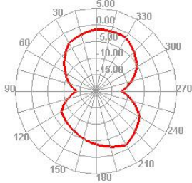
960.000MHz E2
