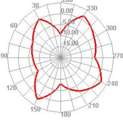
1840.000MHz E2
