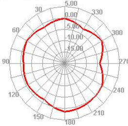
960.000MHz E1
