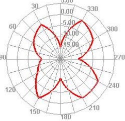
1700.000MHz H
