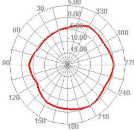
700.000MHz E1
