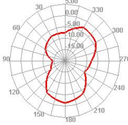
700.000MHz E2
