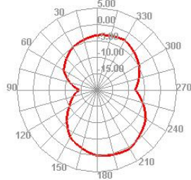
700.000MHz E2
