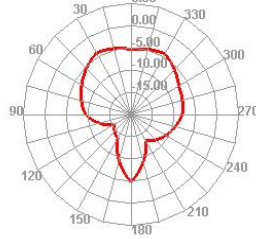
1840.000MHz E1
