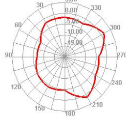
1840.000MHz E2
