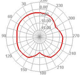
2600.000MHz E1
