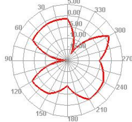
2600.000MHz E2
