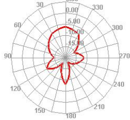
1700.000MHz E1
