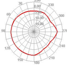
830.000MHz E1
