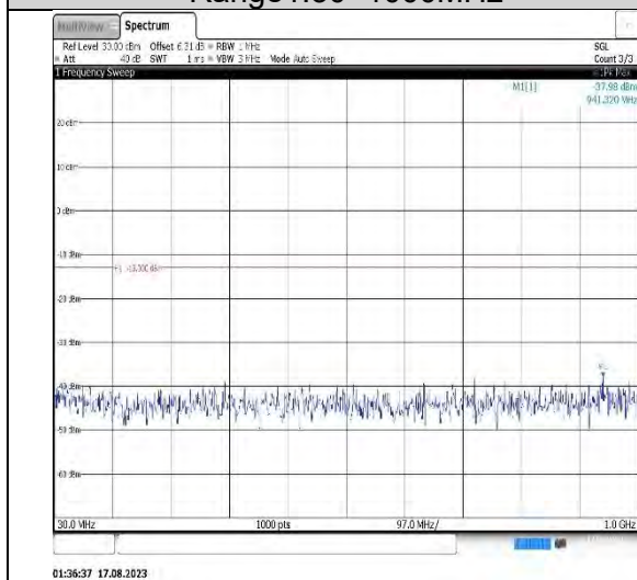
Band25-10MHz-QPSK-26365-1RB#0-Range1:30~1000MHz
