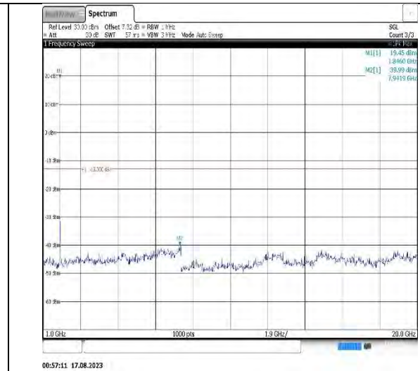
Band25-5MHz-QPSK-26365-1RB#0-Range2:1000~20000MHz
