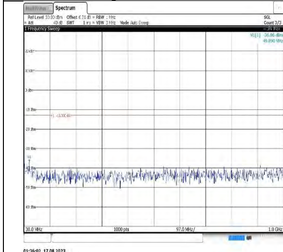
Band25-10MHz-QPSK-26365-1RB#0-Range1:30~1000MHz
