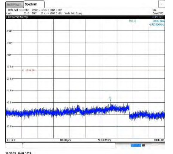
Band12-5MHz-QPSK-23155-1RB#0- Range2:1000~10000MHz
