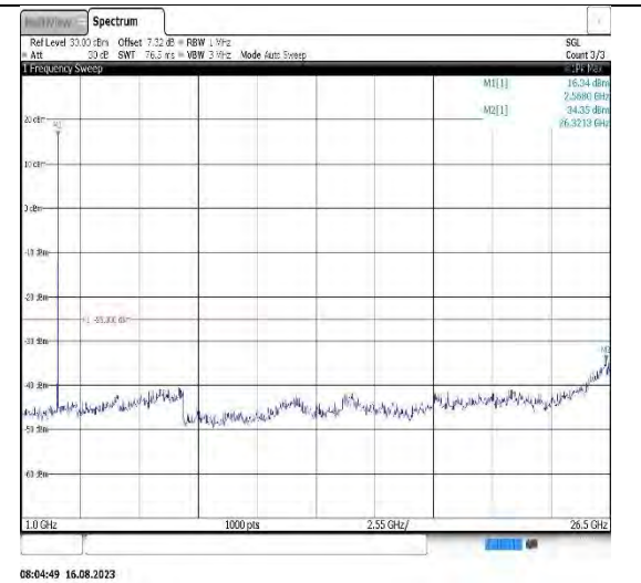
Band7-15MHz-QPSK-20825-1RB#0-Range2:1000~26500MHz
