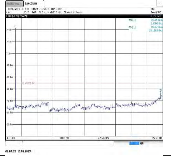
Band7-10MHz-QPSK-21400-1RB#0-Range2:1000~26500MHz
