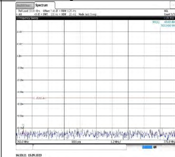
16:33:21 15.09.2023 Band 13-5MHz-QPSK-23205-1RB#0-Range2:763~775MHz
