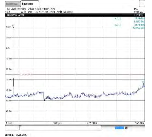
Band7-20MHz-16QAM-21350-1RB#0-Range2:1000~26500MHz
