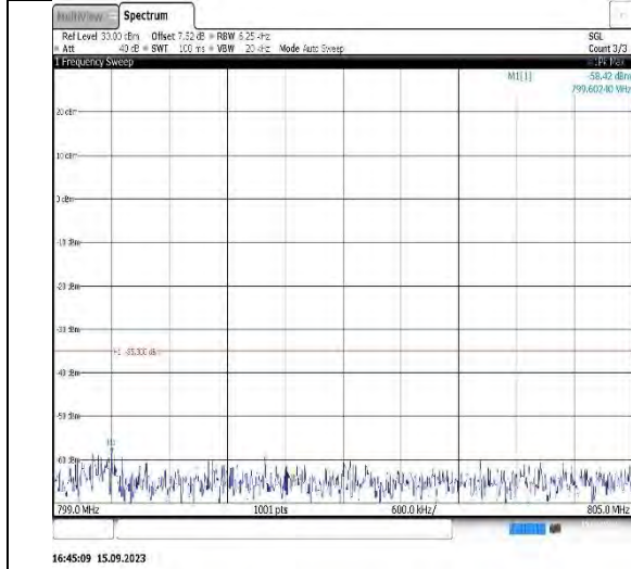
Band14-5MHz-QPSK-23330-1RB#0- Range3:799~805MHz
