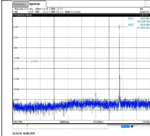
Band13-5MHz-QPSK-23255-1RB#0-Range1:30~1000MHz
