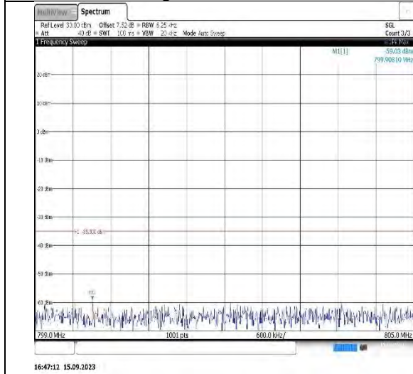
Band14-10MHz-QPSK-23330-1RB#0- Range3:799~805MHz
