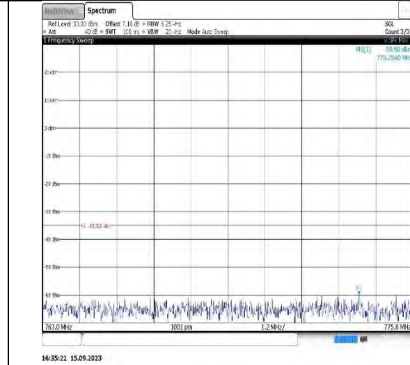
Band13-5MHz-QPSK-23255-1RB#0-Range2:763~775MHz
