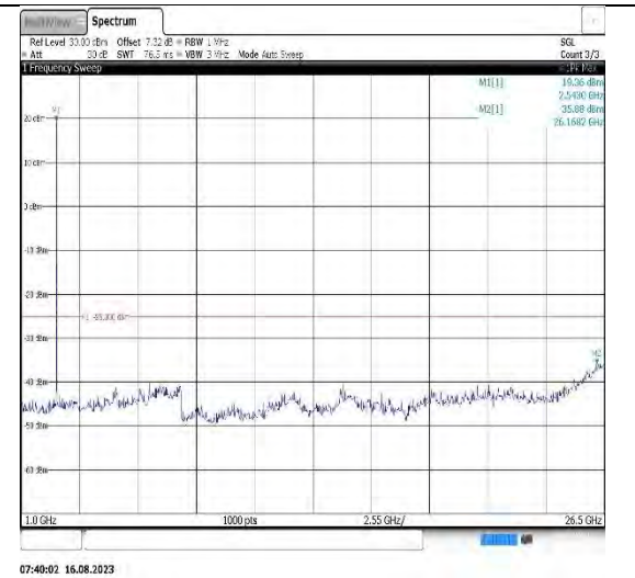
Band7-5MHz-QPSK-21425-1RB#0-Range2:1000~26500MHz
