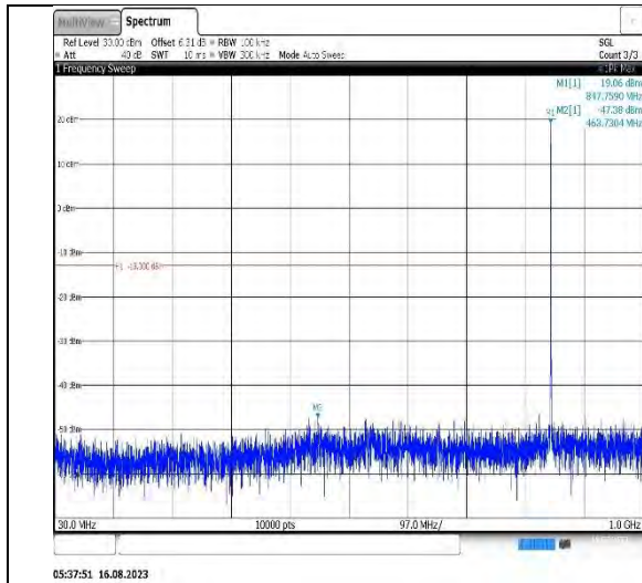
Band5-3MHz-QPSK-20415-1RB#0- Range1:30~1000MHz
