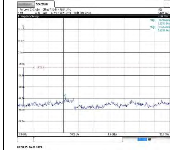
Band4-3MHz-QPSK-20385-1RB#0- Range2:1000~20000MHz
