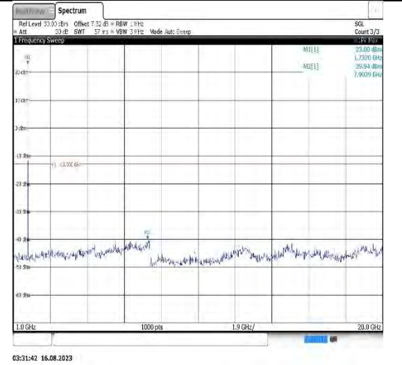
Band4-5MHz-QPSK-19975-1RB#0-Range2:1000~20000MHz
