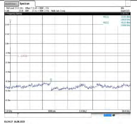
Band2-20MHz-16QAM-18900-1RB#0- Range2:1000~20000MHz
