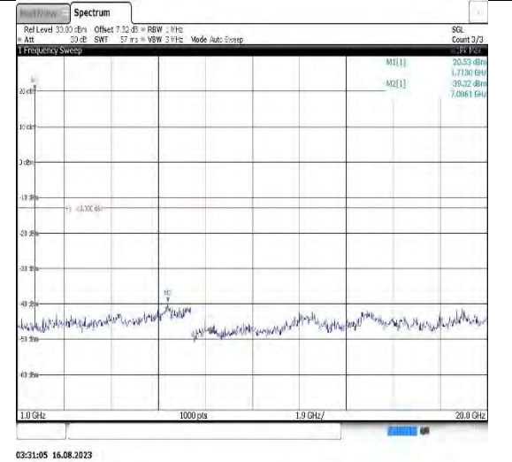
Band4-5MHz-QPSK-20175-1RB#0-Range2:1000~20000MHz
