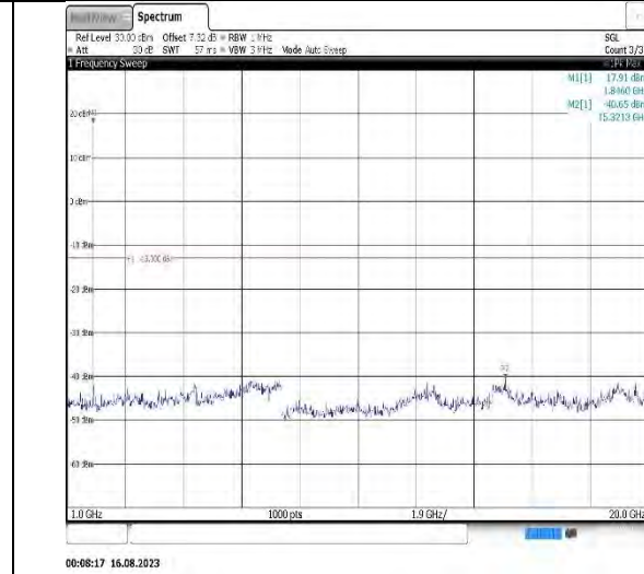
Band2-3MHz-16QAM-18615-1RB#0-Range2:1000~20000MHz
