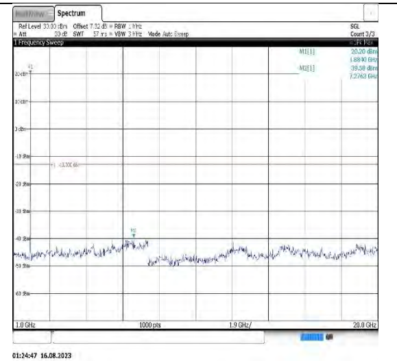
Band2-20MHz-16QAM-18700-1RB#0- Range2:1000~20000MHz
