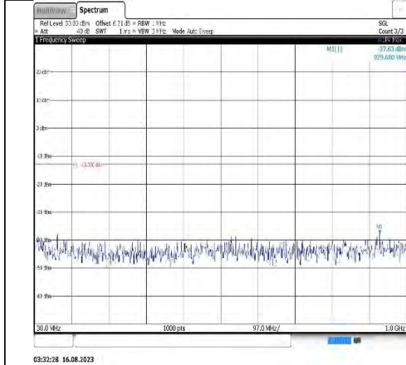
Band4-10MHz-QPSK-20000-1RB#0-Range1:30~1000MHz
