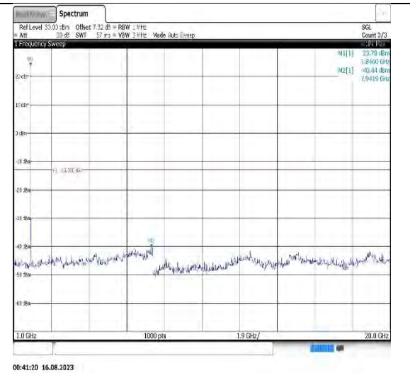
Band2-5MHz-QPSK-18900-1RB#0-Range2:1000~20000MHz
