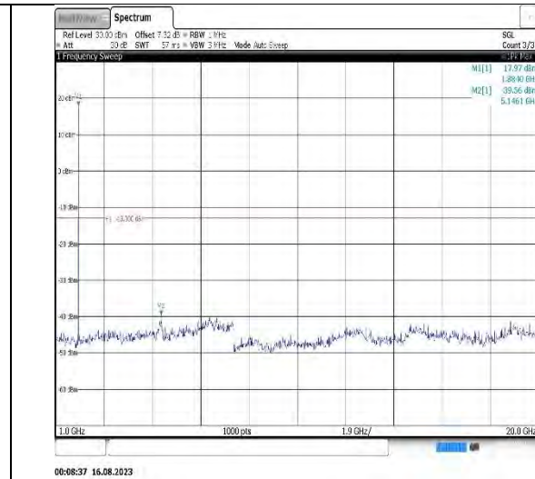
Band2-3MHz-QPSK-19185-1RB#0-Range2:1000~20000MHz
