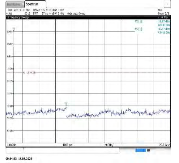
Band2-10MHz-QPSK-18900-1RB#0-Range2:1000~20000MHz
