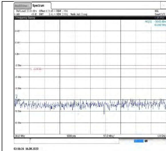
Band4-1.4MHz-QPSK-20393-1RB#0-Range1:30~1000MHz
