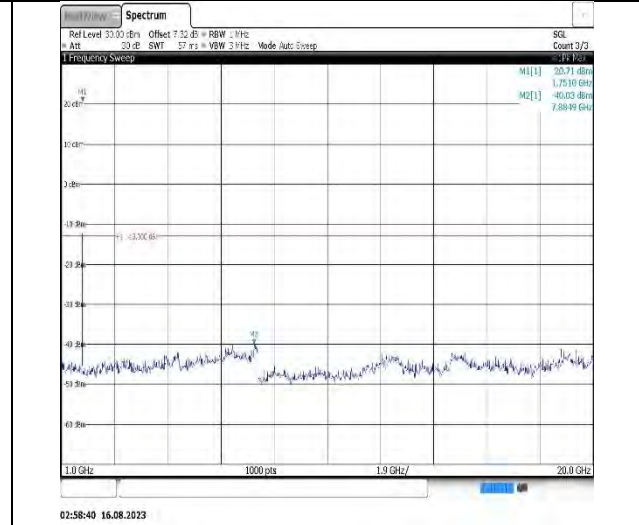
Band4-3MHz-QPSK-20175-1RB#0- Range2:1000~20000MHz
