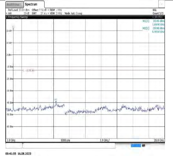
Band2-5MHz-QPSK-19175-1RB#0-Range2:1000~20000MHz
