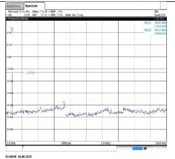
Band4-5MHz-QPSK-19975-1RB#0-Range2:1000~20000MHz
