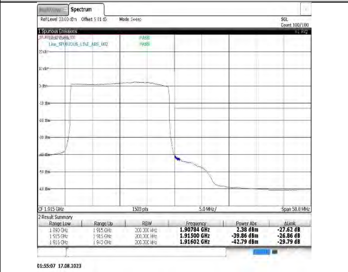
Band25-20MHz-QPSK-26590-100RB#0
