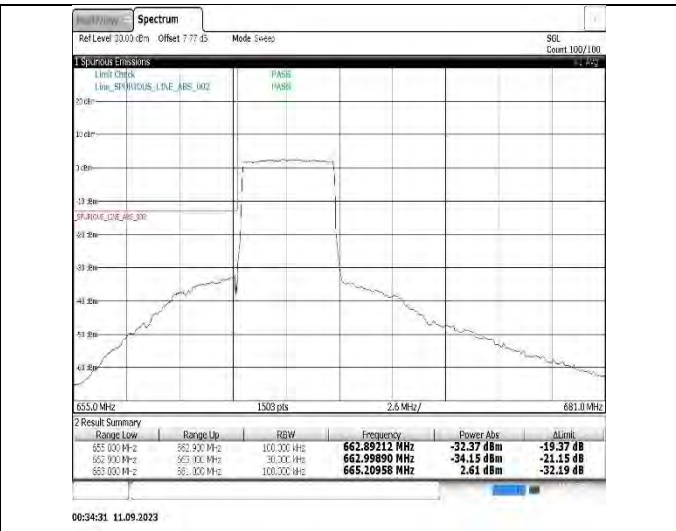
Band71-10MHz-QPSK-133172-50RB#0
