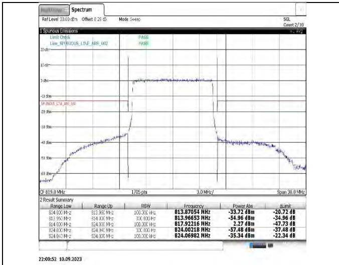
Band26(824-849)-10MHz-QPSK-26990-50RB#0
