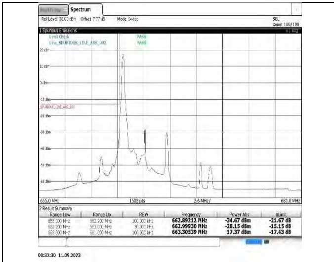
Band71-10MHz-QPSK-133172-1RB#0
