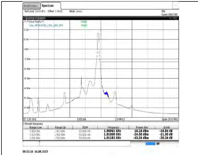
Band2-5MHz-16QAM-18625-1RB#0
