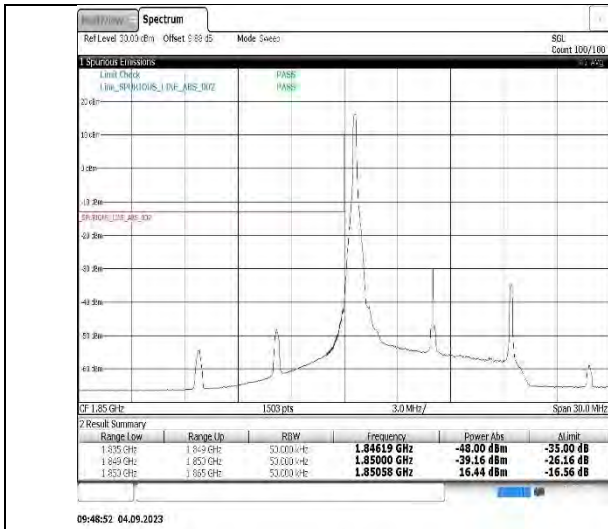
Band2-10MHz-QPSK-18650-50RB#0
