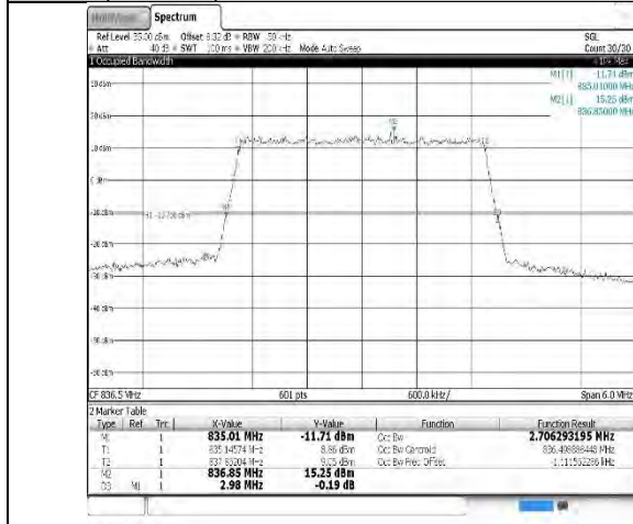
10:07:58 24.08.2023 B26(824-849)-5MHz-QPSK-26915-25RB#0-PASS
