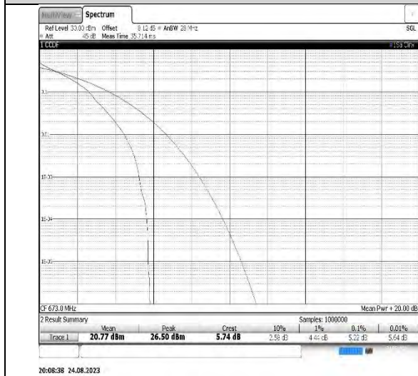
Band71-20MHz-QPSK-133322-1RB#0
