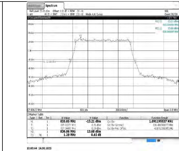
10:00:44 24.08.2023 B26(824-849)-3MHz-16QAM-26915-15RB#0-PASS
