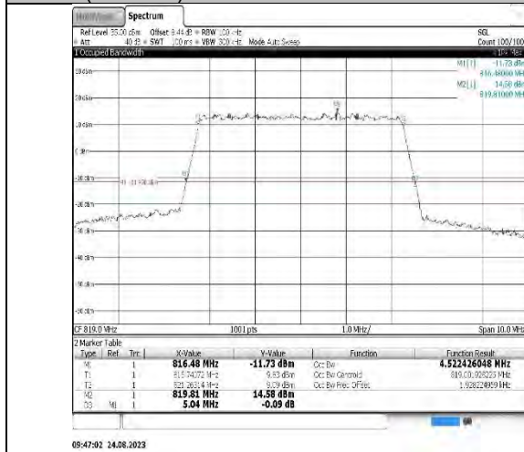
B26(814-824)-10MHz-QPSK-26740-50RB#0-PASS
