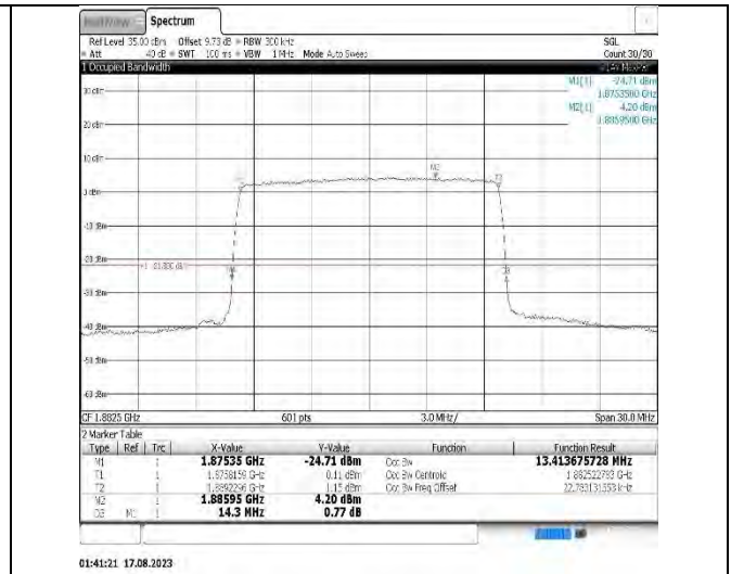
Band25-20MHz-16QAM-26365-100RB#0
