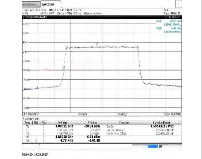
Band25-10MHz-16QAM-26365-50RB#0
