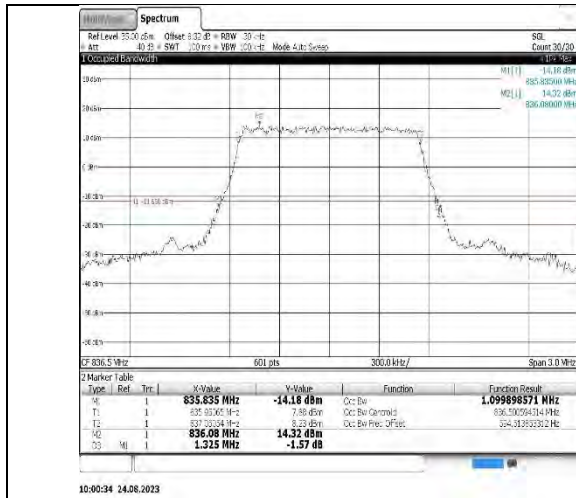
10:00:34 24.08.2023 B26(824-849)-3MHz-QPSK-26915-15RB#0-PASS
