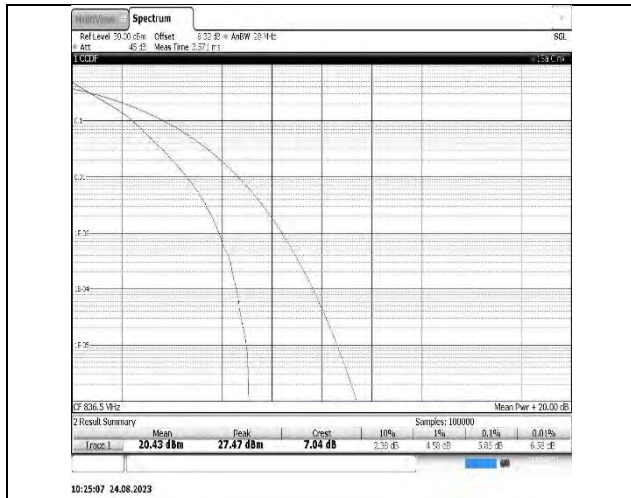
B26(824-849)-10MHz-QPSK-26915-50RB#0-PASS
