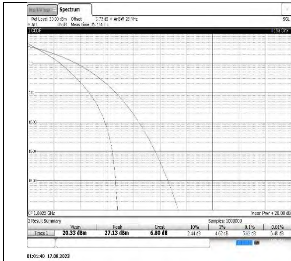
Band25-10MHz-QPSK-26365-50RB#0
