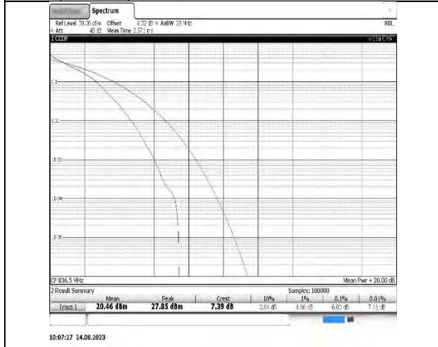
B26(824-849)-3MHz-QPSK-26915-15RB#0-PASS
