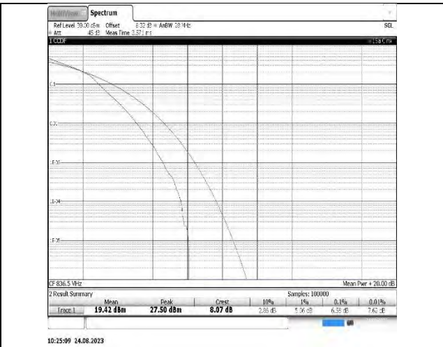
B26(824-849)-10MHz-16QAM-26915-50RB#0-PASS
