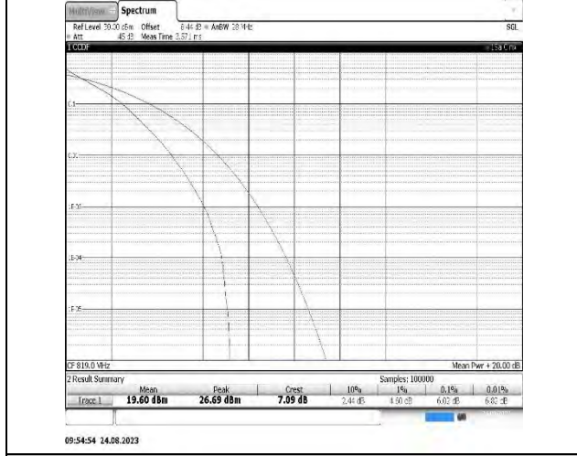
B26(814-824)-10MHz-QPSK-26740-50RB#0-PASS
