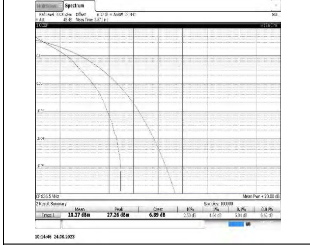
B26(824-849)-5MHz-QPSK-26915-25RB#0-PASS
