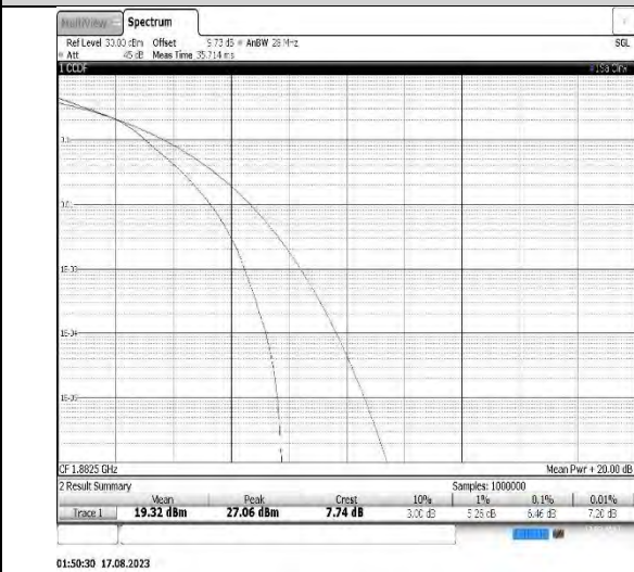
Band25-20MHz-16QAM-26365-100RB#0
