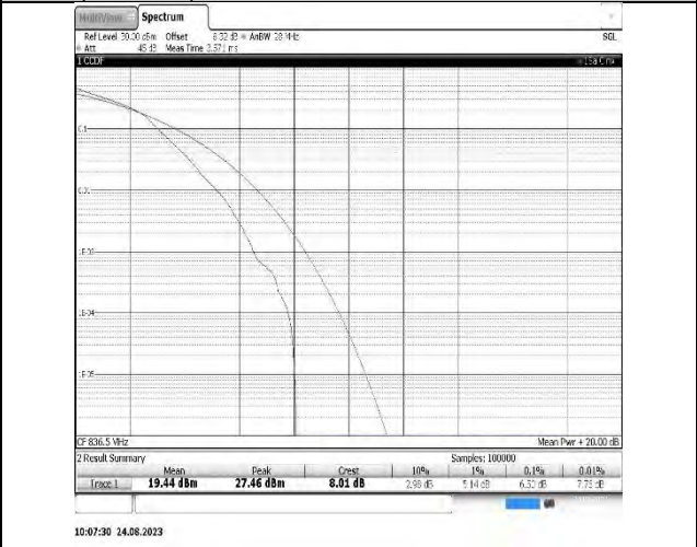
B26(824-849)-3MHz-16QAM-26915-15RB#0-PASS
