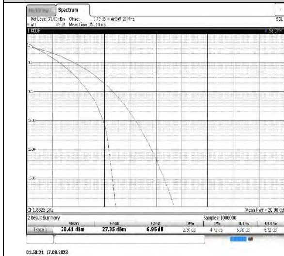
Band25-20MHz-QPSK-26365-100RB#0
