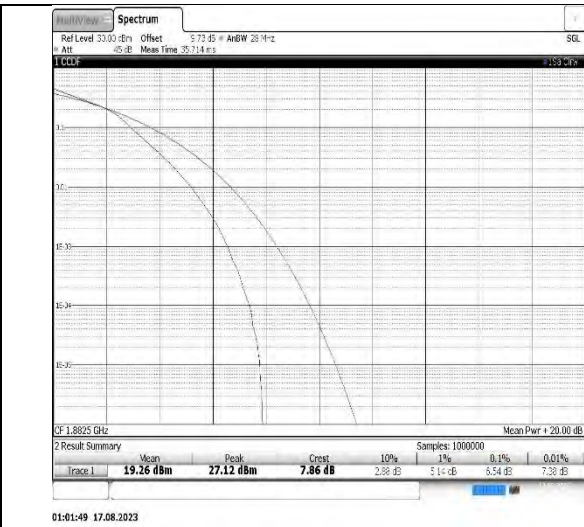
Band25-10MHz-16QAM-26365-50RB#0
