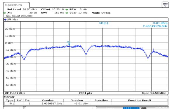
b_2437MHz_Chain 0
