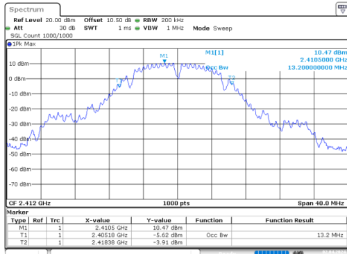
b_2412MHz_Chain 0
