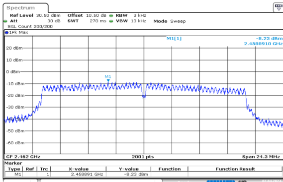
n20_2462MHz_Chain 0
