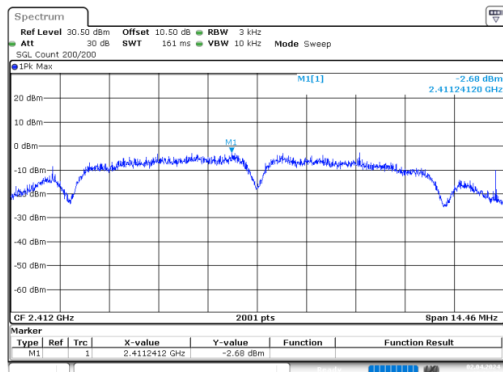
b_2412MHz_Chain 0
