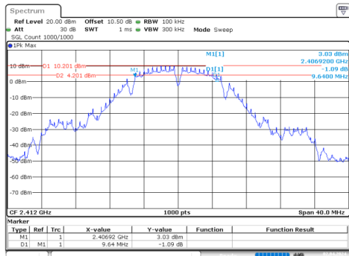
b_2412MHz_Chain 0
