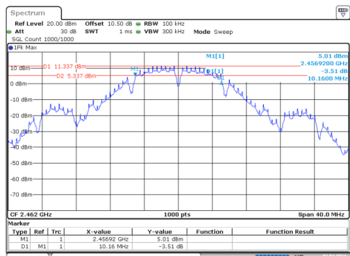
b_2462MHz_Chain 0
