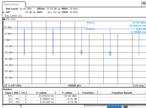
b_2437MHz_Chain 0
