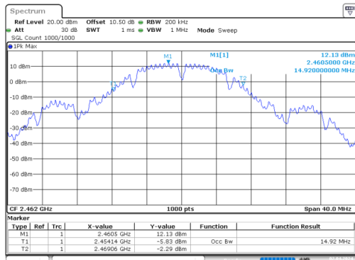
b_2462MHz_Chain 0
