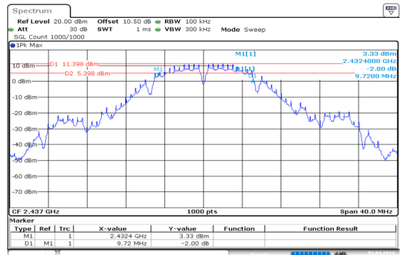
b_2437MHz_Chain 0
