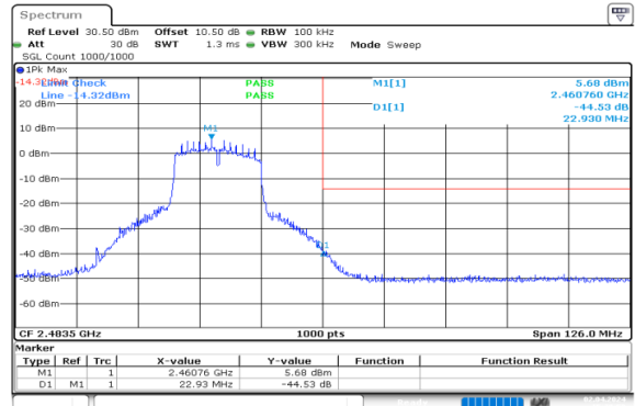
n20_2462MHz_Chain 0
