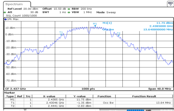
b_2437MHz_Chain 0
