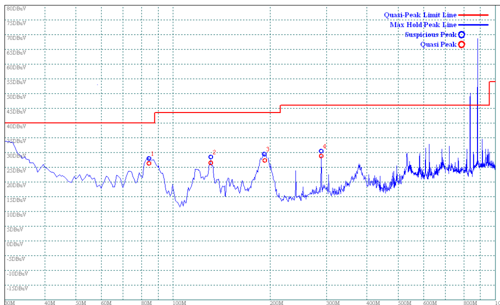
(Plot A: Test Antenna Vertical)
