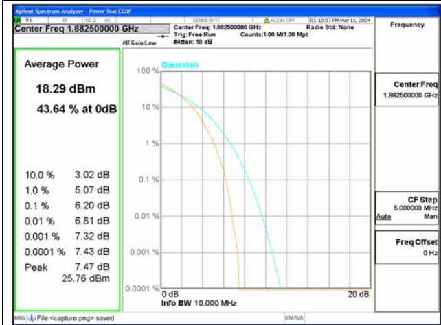
B25 / 10MHz / Mid CH / 64QAM
